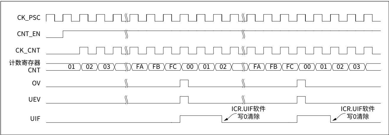
图 11-3 连续计数模式示例
