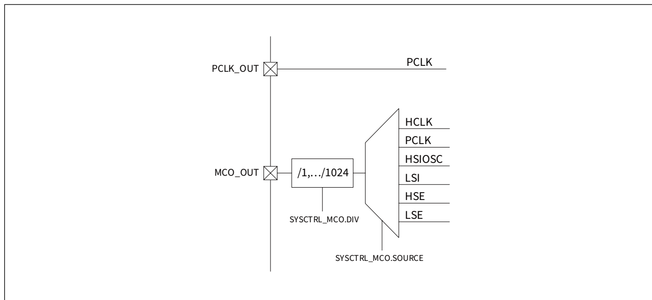
图 4-5 时钟输出
