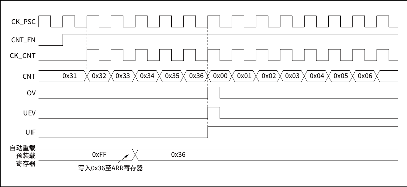
图 13-8 递增计数，当重载缓存使能时的更新事件（GTIM_CR1.ARPE=1）
