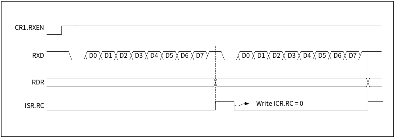
图 16-6 异步工作模式接收控制时序（接收两个字数据）
