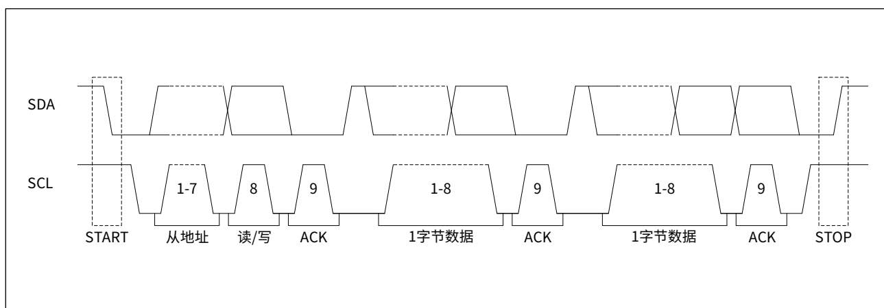
图 18-1 I2C 协议帧
