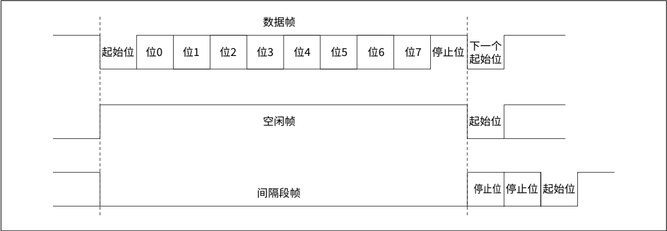
图 16-5 间隔段帧和空闲帧时序
