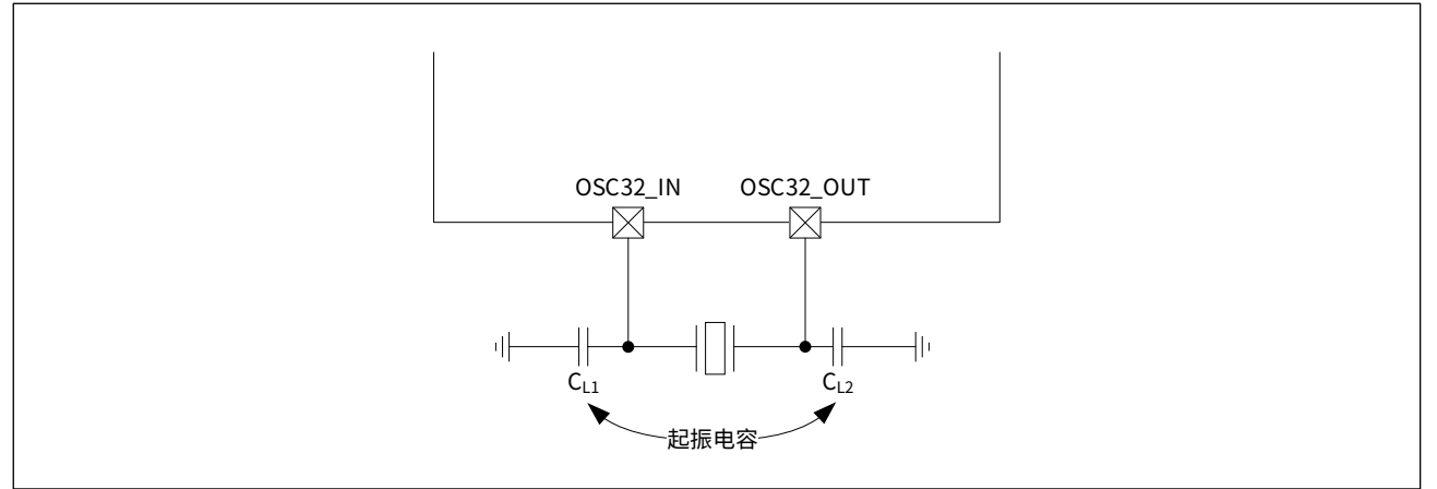
图 4-3 LSE 外接石英晶体 / 陶瓷谐振器连接方式
