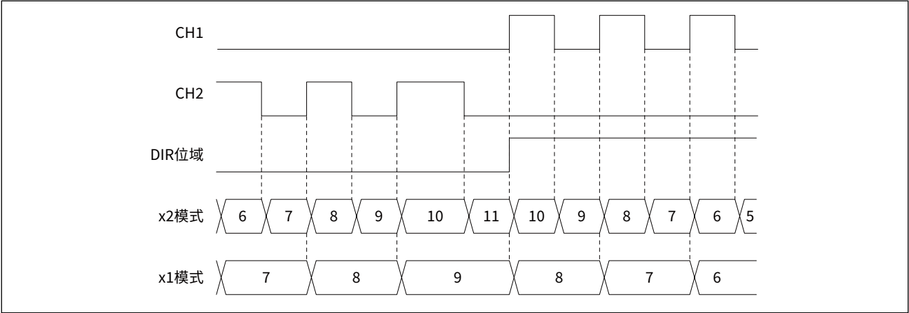
图 13-32 定向时钟编码器模式计数示例 (CC1P = CC2P = 1)
