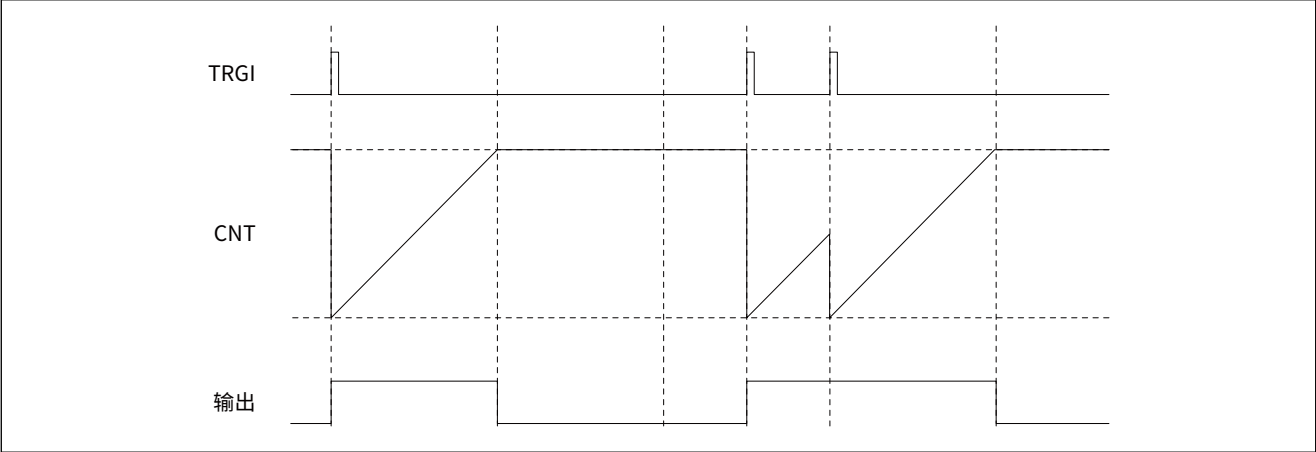
图 14-52 可再触发单脉冲模式 2 示例
