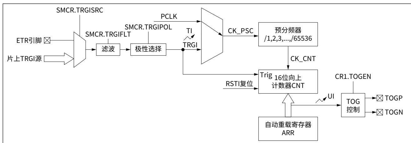
图 11-7 触发启动模式框图
