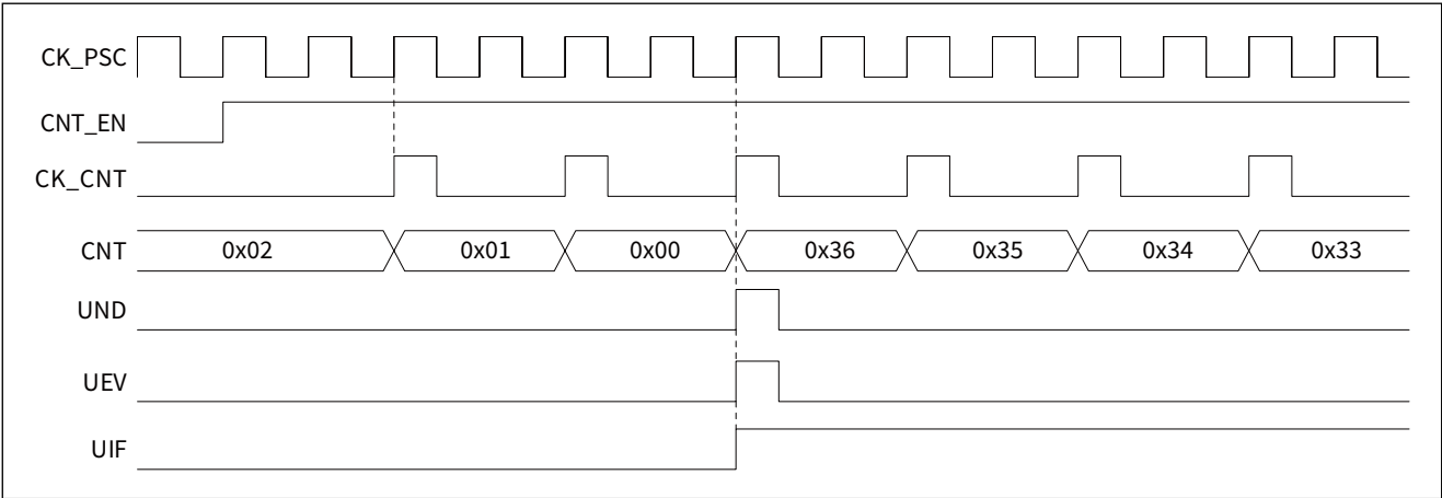
图 14-11 递减计数，内部时钟分频因子为 4
