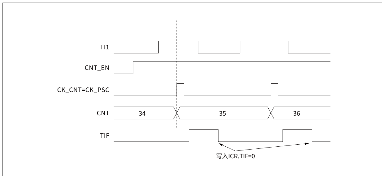
图 14-23 外部时钟模式 1 时序示例
