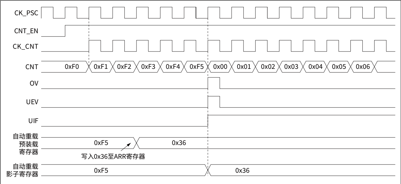
图 13-8 递增计数，当重载缓存使能时的更新事件（GTIMx_CR1.ARPE=1）
