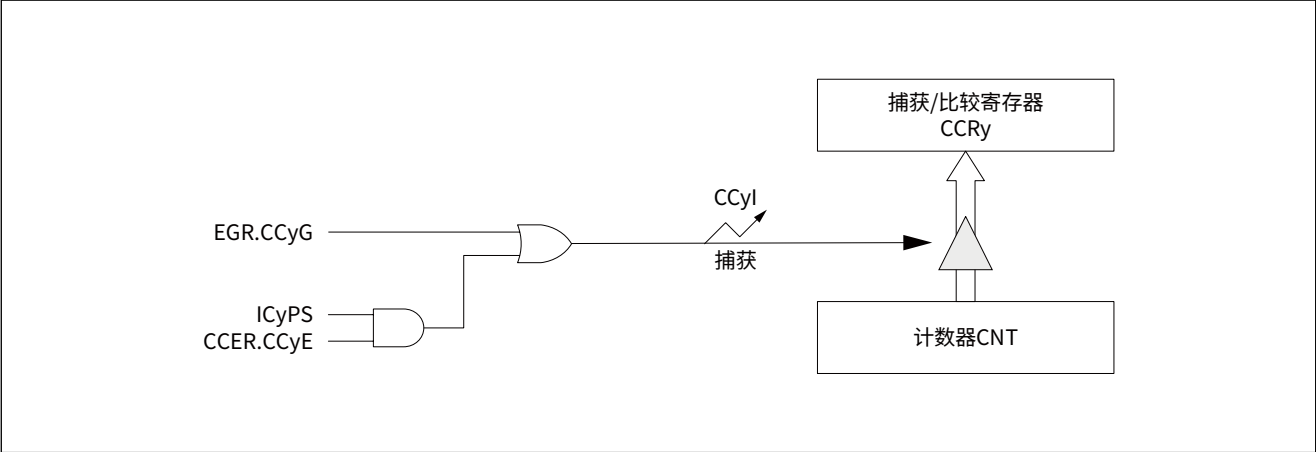
图 14-34 输入捕获模式框图
