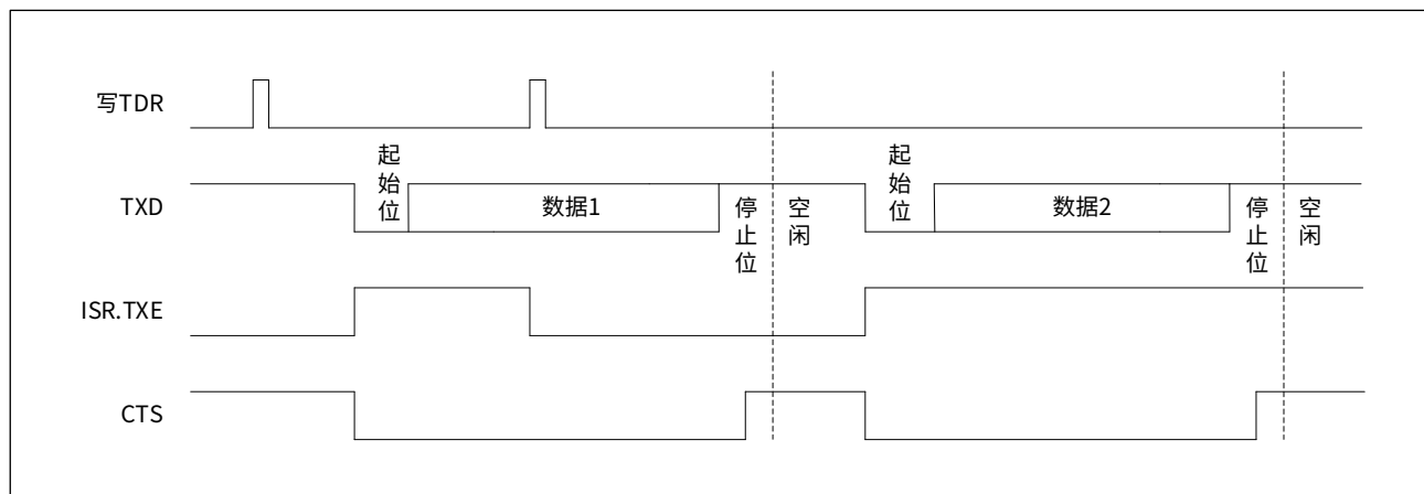
图 16-9 CTS 流控时序
