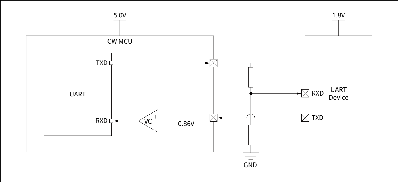
图 16-11 不同电压器件通信示意图
