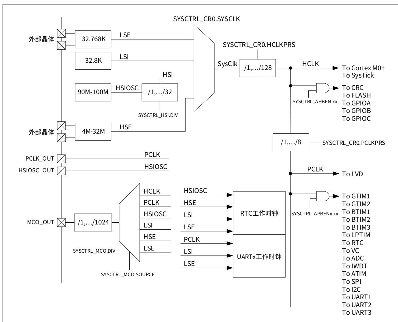
图 4-1 系统内部时钟树
