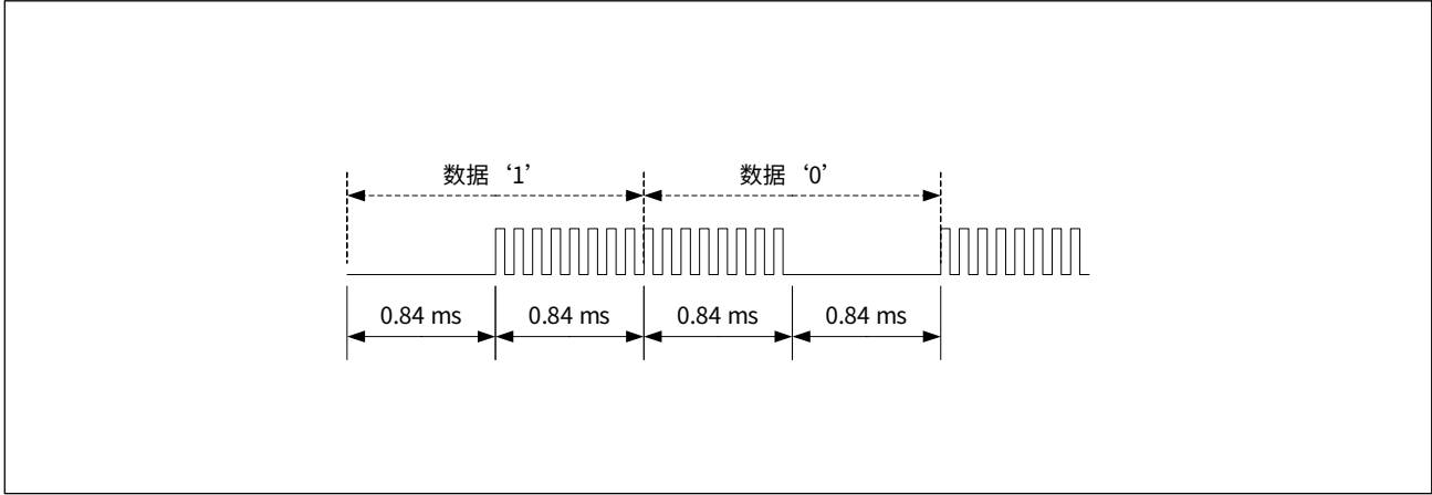
图 19-2 PPM 调制方式
