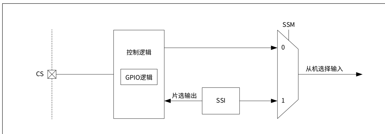
图 17-3 从机选择引脚管理
