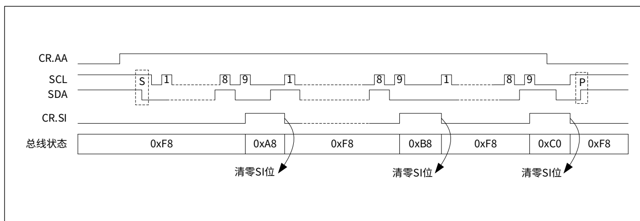
图 18-14 从机发送模式状态同步图
