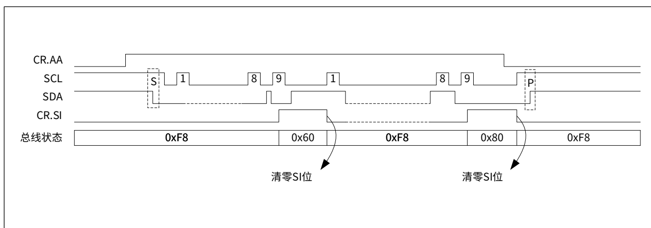
图 18-12 从机接收模式状态同步图
