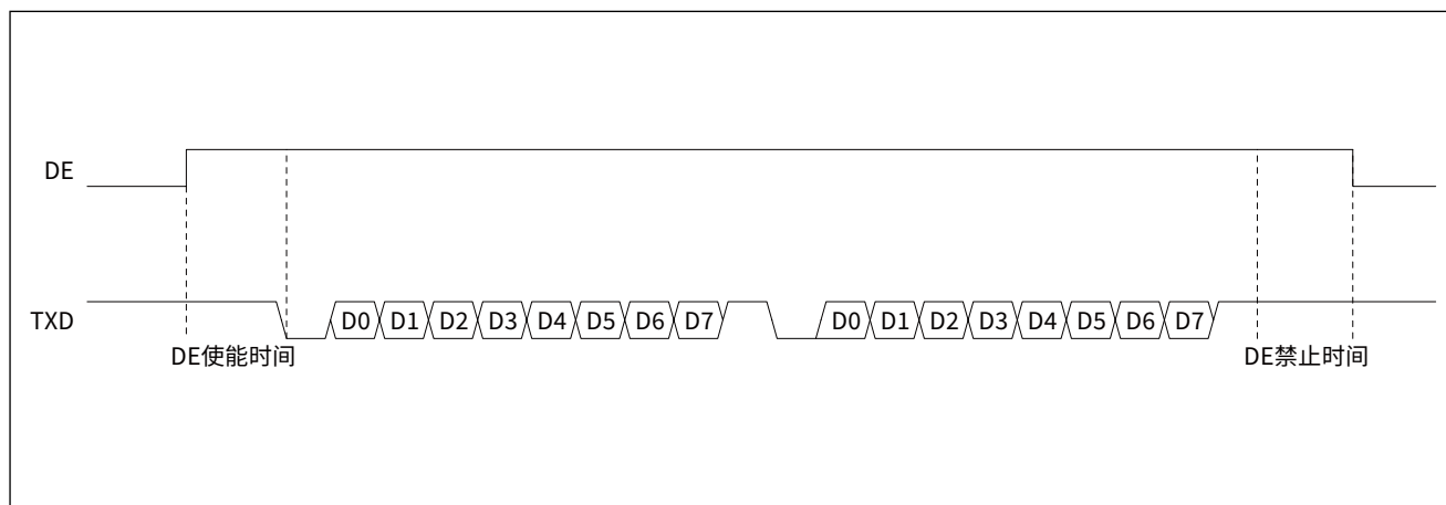
图 16-10 驱动器使能时序
