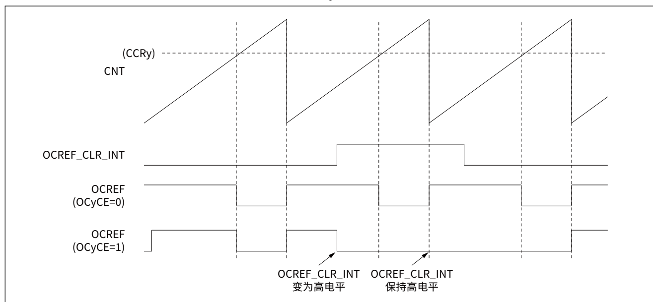
图 13-45 OCyREF 清零示例
