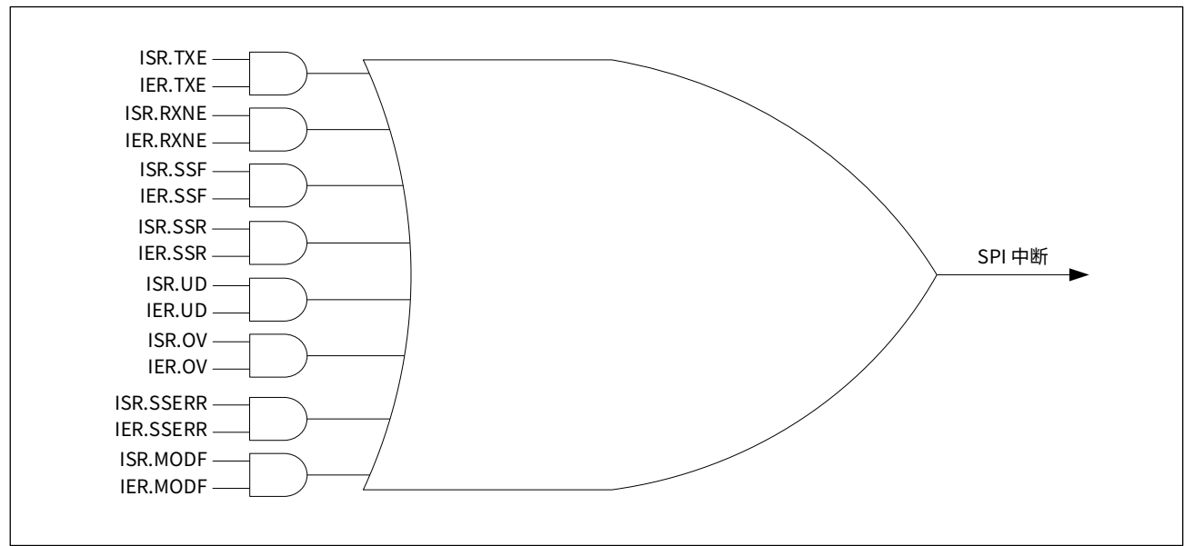
图 17-11 SPI 中断
