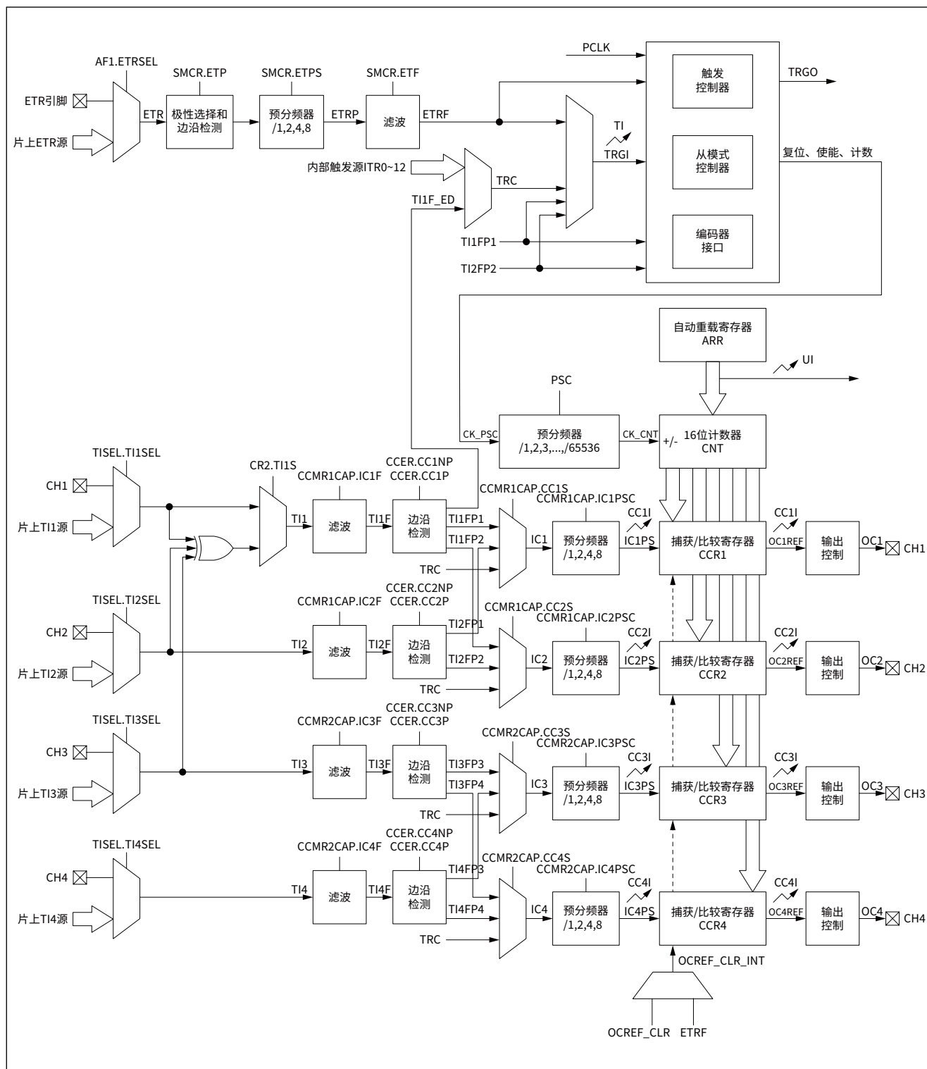
图 13-1 GTIM 功能框图
