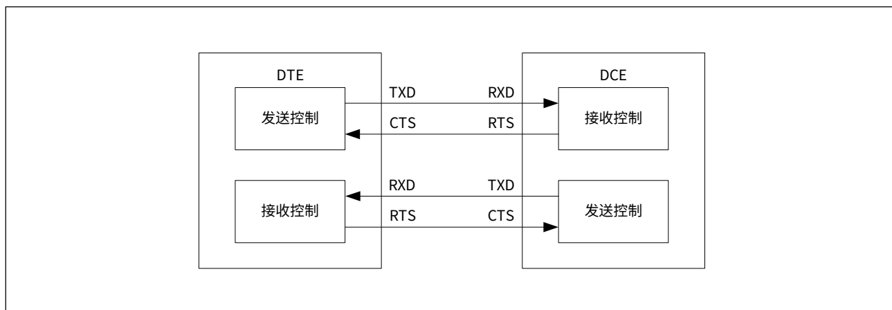
图 16-7 硬件流控示意图
