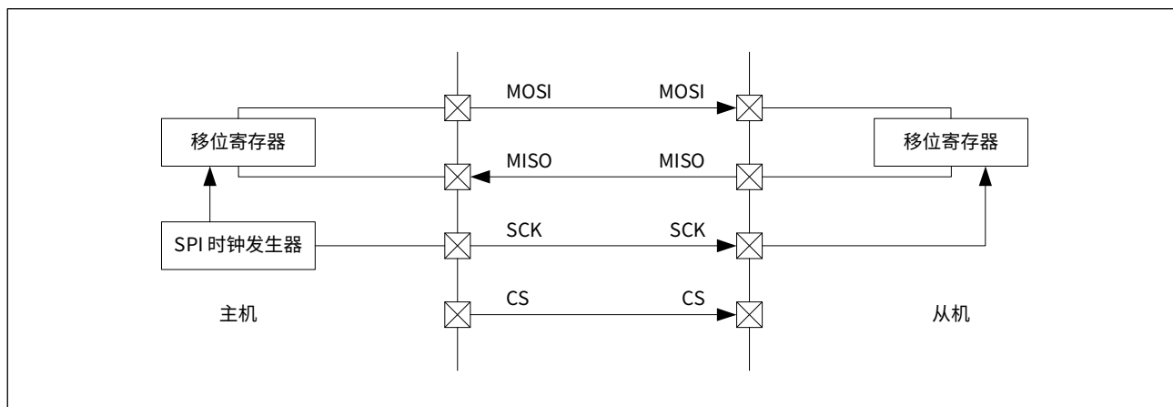
图 17-4 全双工通信模式
