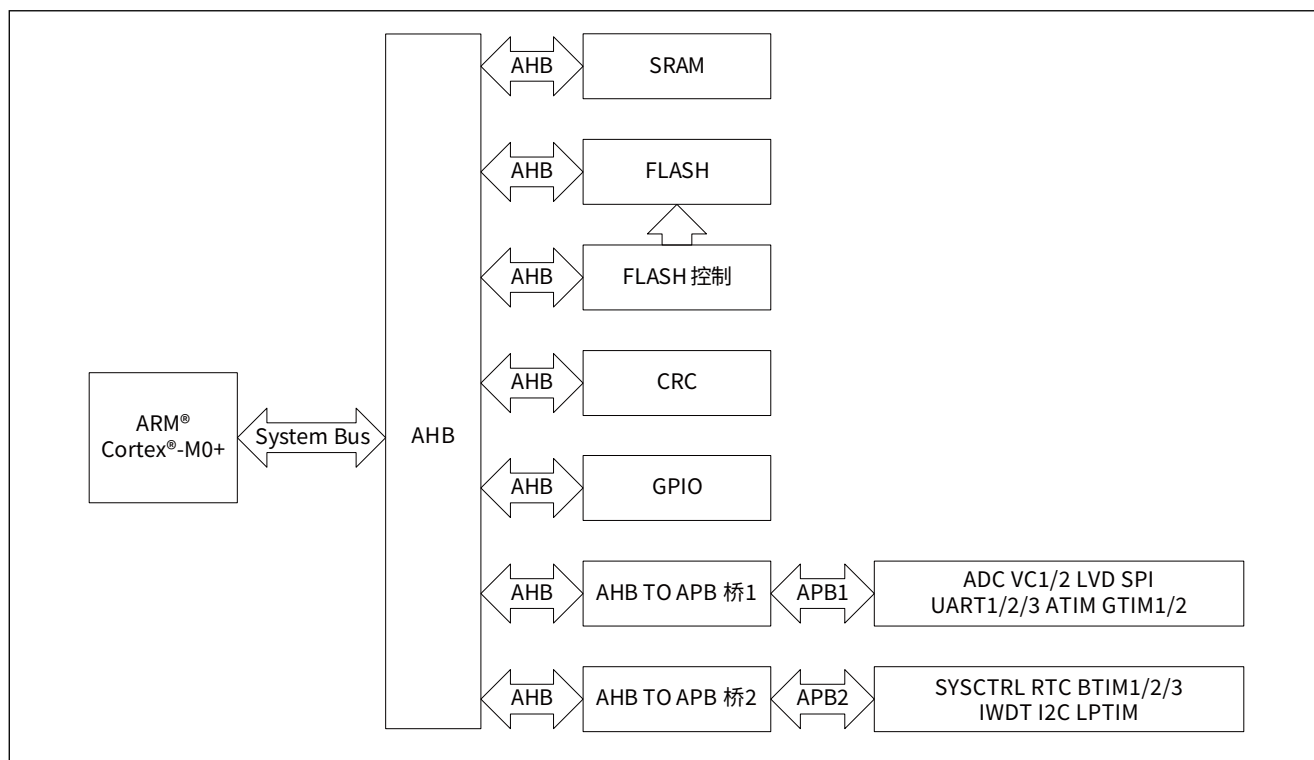
图 2-1 系统架构
