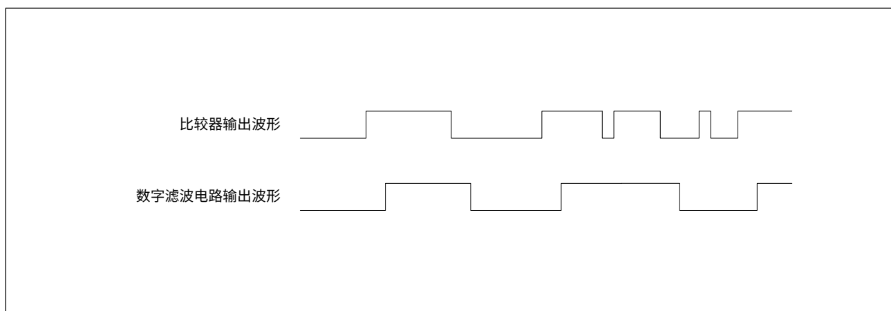
图 21-2 VC 滤波响应时间
