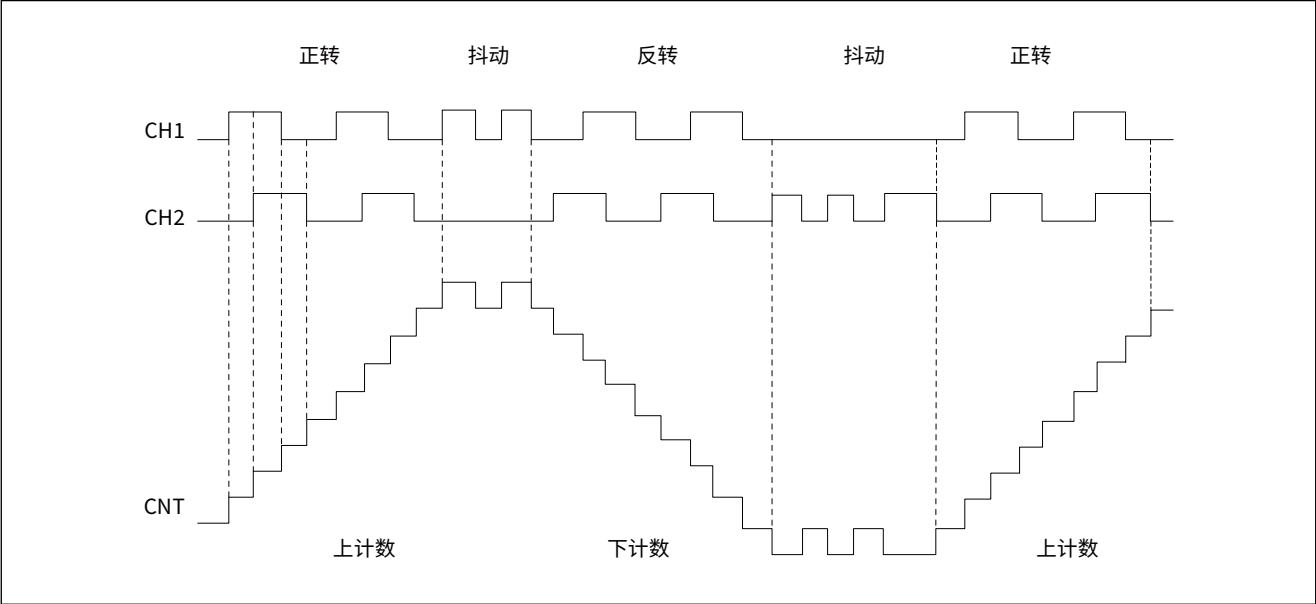
图 13-28 正交编码器模式 -x4 模式操作示例
