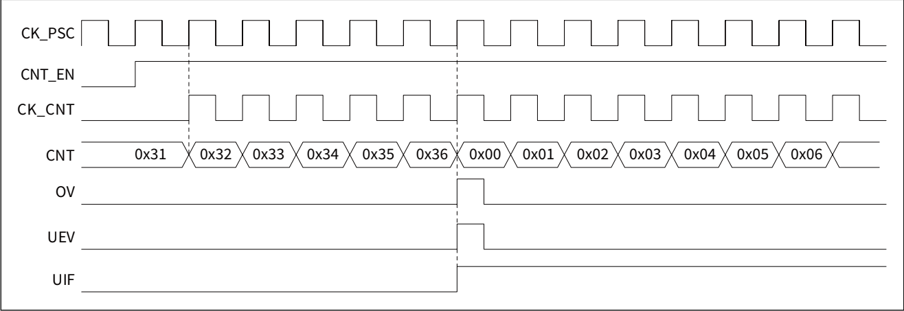
图 14-3 递增计数，内部时钟分频因子为 1
