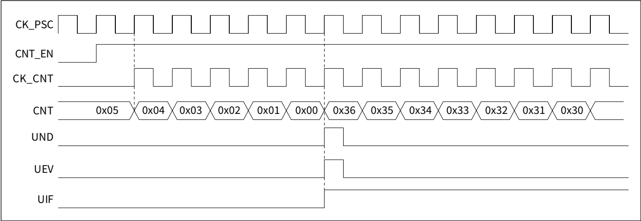
图 14-10 递减计数，内部时钟分频因子为 2
