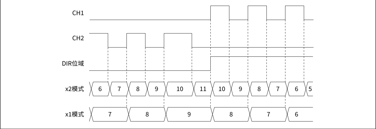
图 14-33 定向时钟编码器模式计数示例 (CC1P = CC2P = 1)
