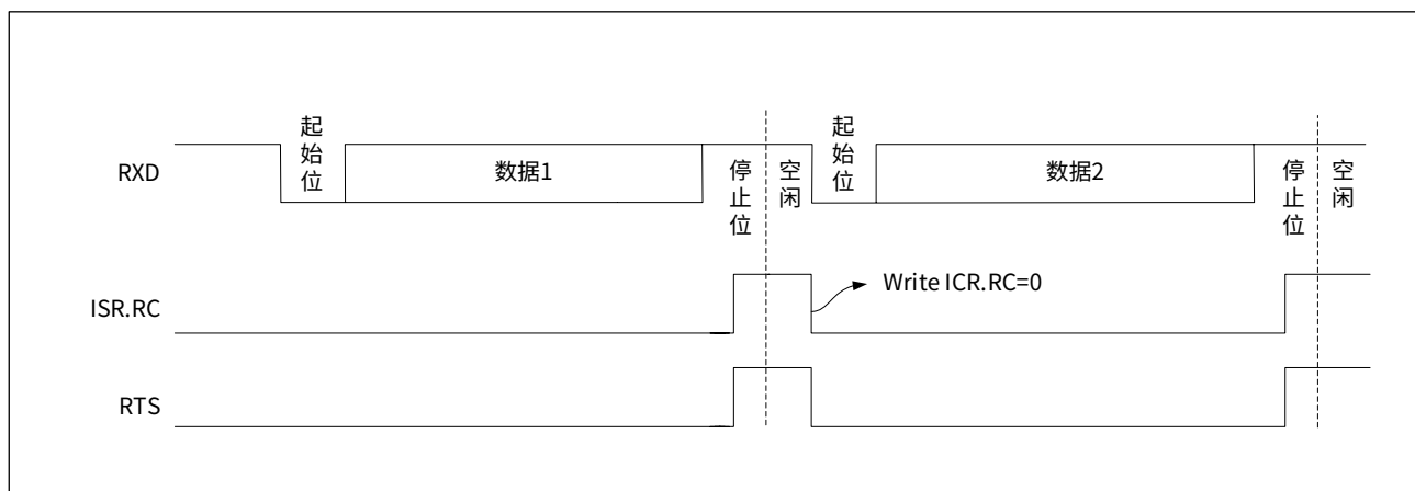
图 16-8 RTS 流控时序
