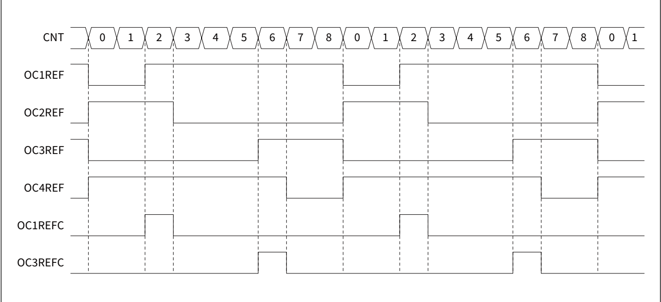
图 13-43 组合 PWM 模式 2 示例
