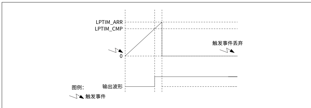
图 12-4 LPTIM 单次置位波形
