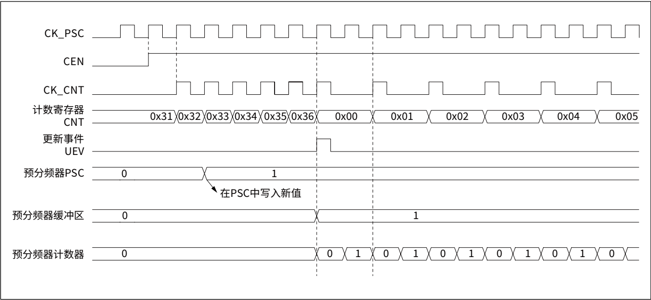
图 13-2 预分频器分频由 1 变为 2 时的时序图
