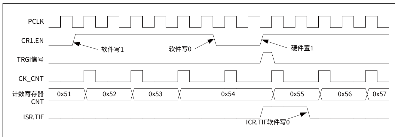
图 11-8 触发启动模式时序图
