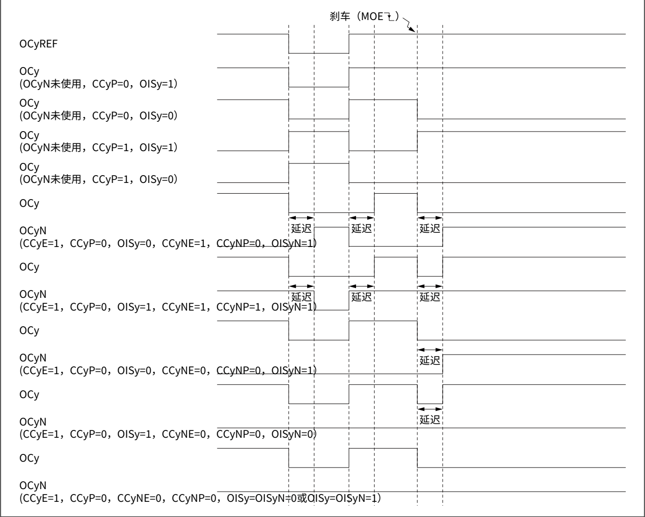
图 14-50 响应刹车事件 BRK 时的输出行为 (OSSI=0)
