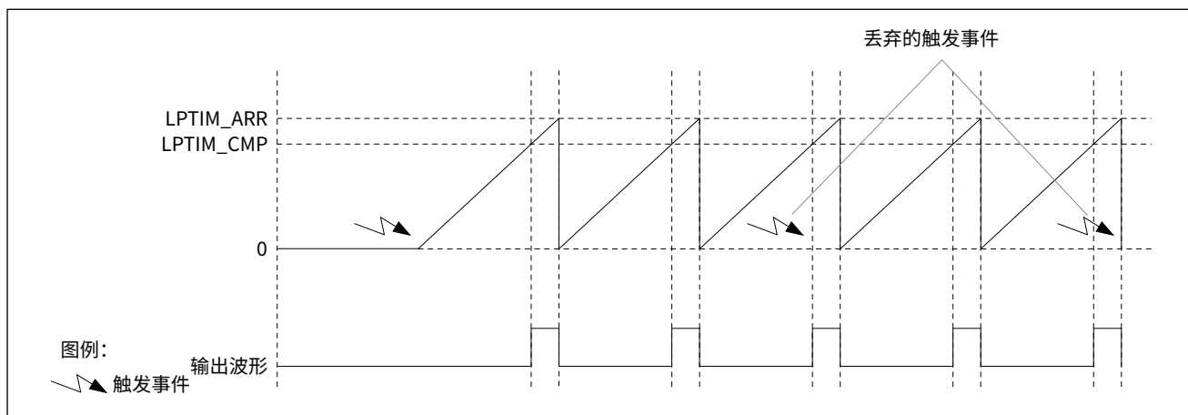
图 12-5 LPTIM 连续模式
