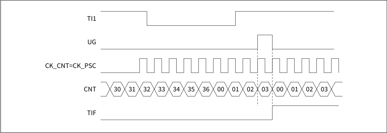
图 14-25 复位模式时序
