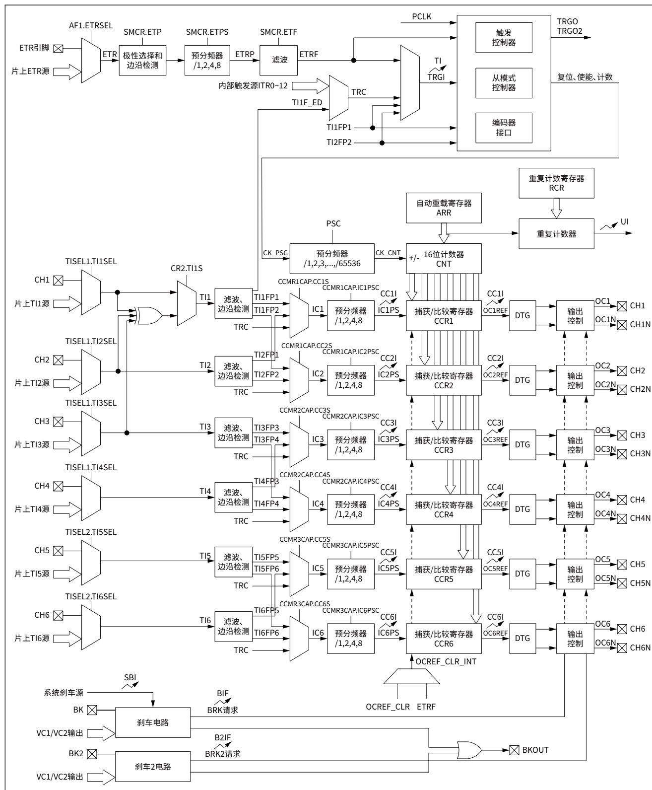
图 14-1 ATIM 功能框图
