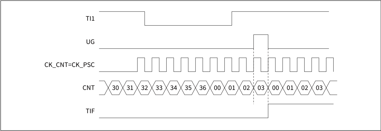
图 13-24 复位模式时序
