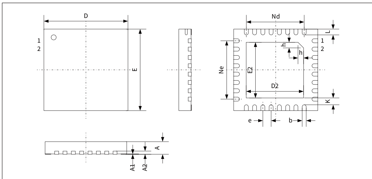
图 8-3 QFN32 引线
