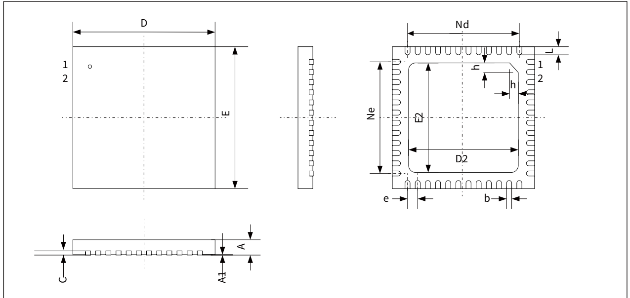
图 8-1 QFN48 引线
