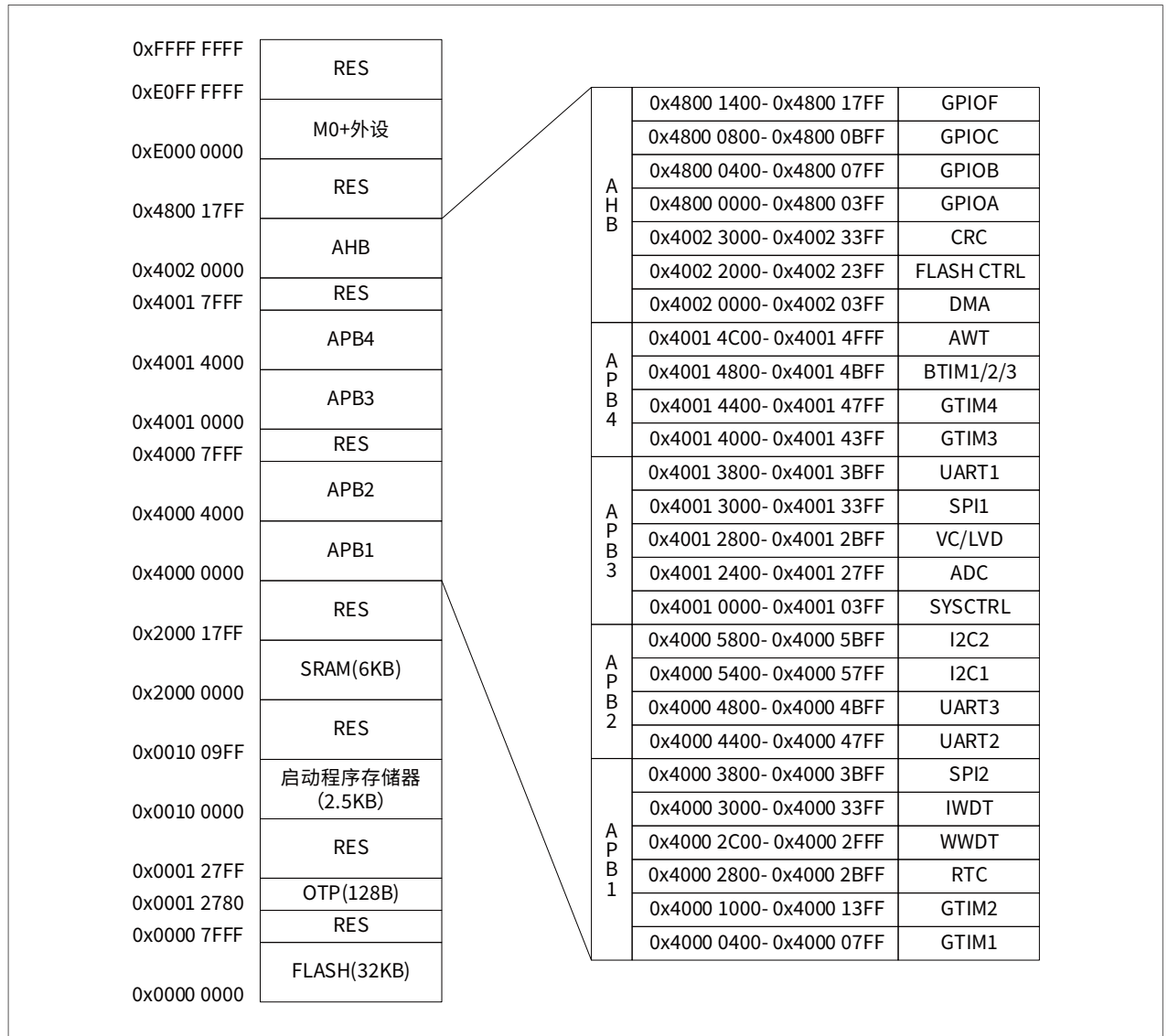
图 6-1 CW32F020 的内部地址镜像
