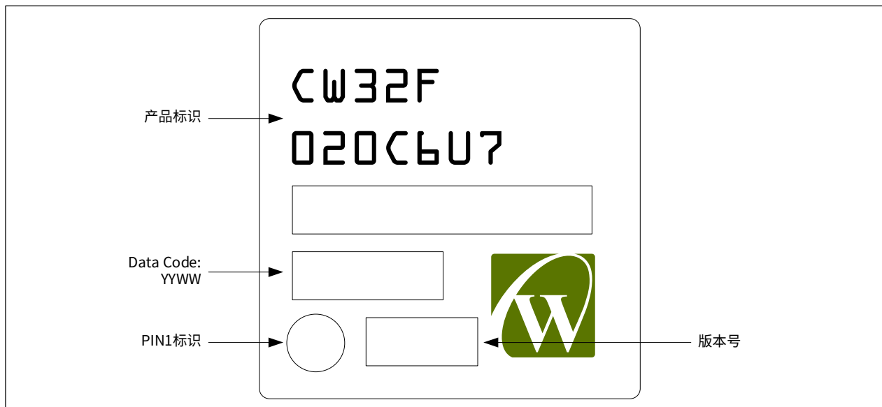
图 8-2 QFN48 顶部标记示例
