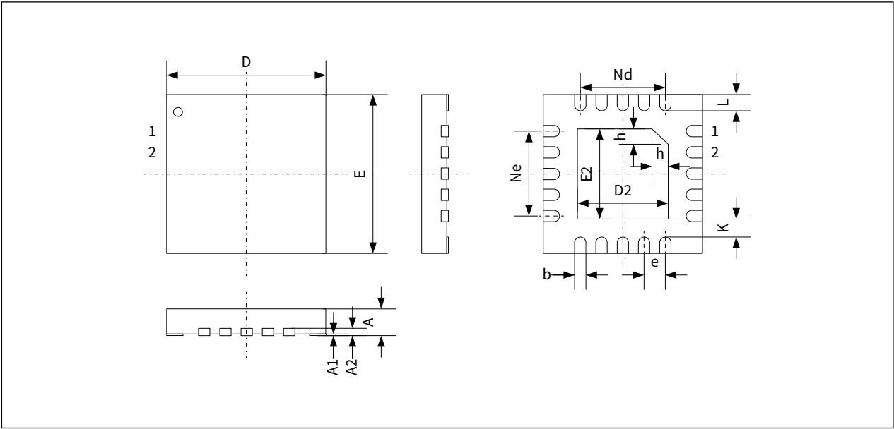
图 8-5 QFN20 引线
