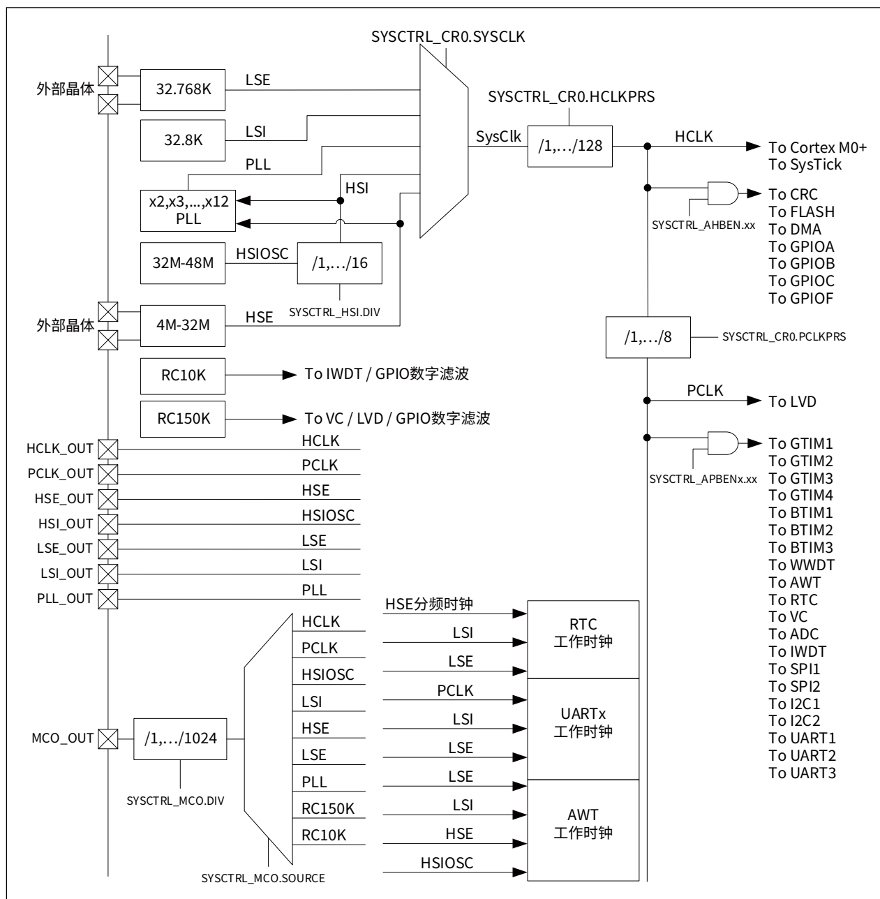
图 4-1 CW32F020 的时钟树
