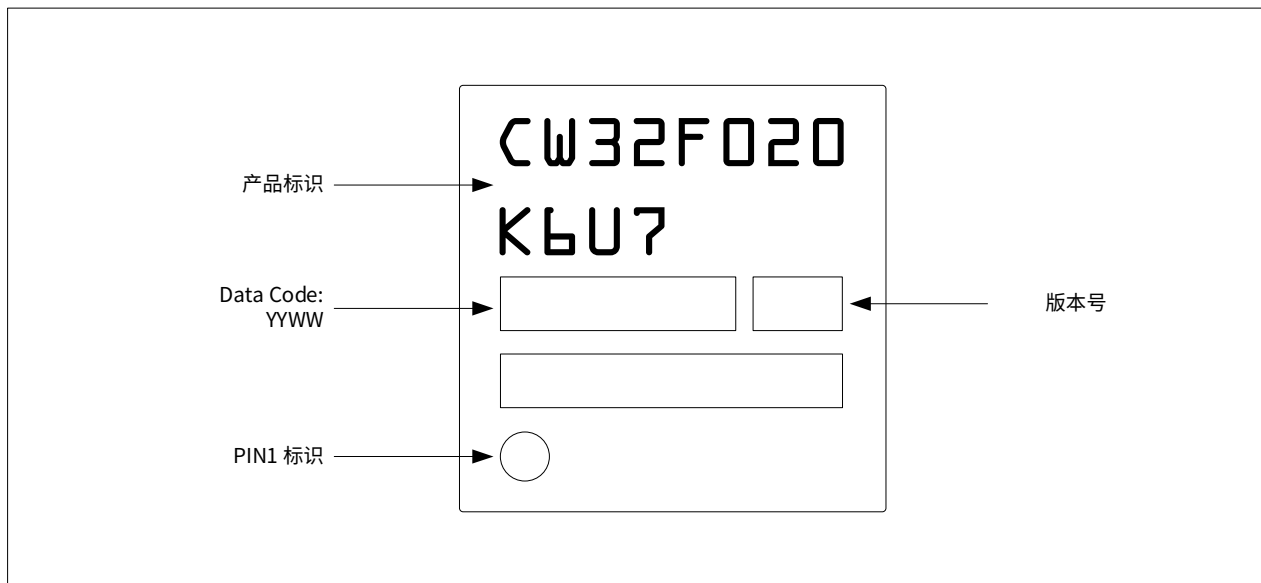
图 8-4 QFN32 顶部标记示例
