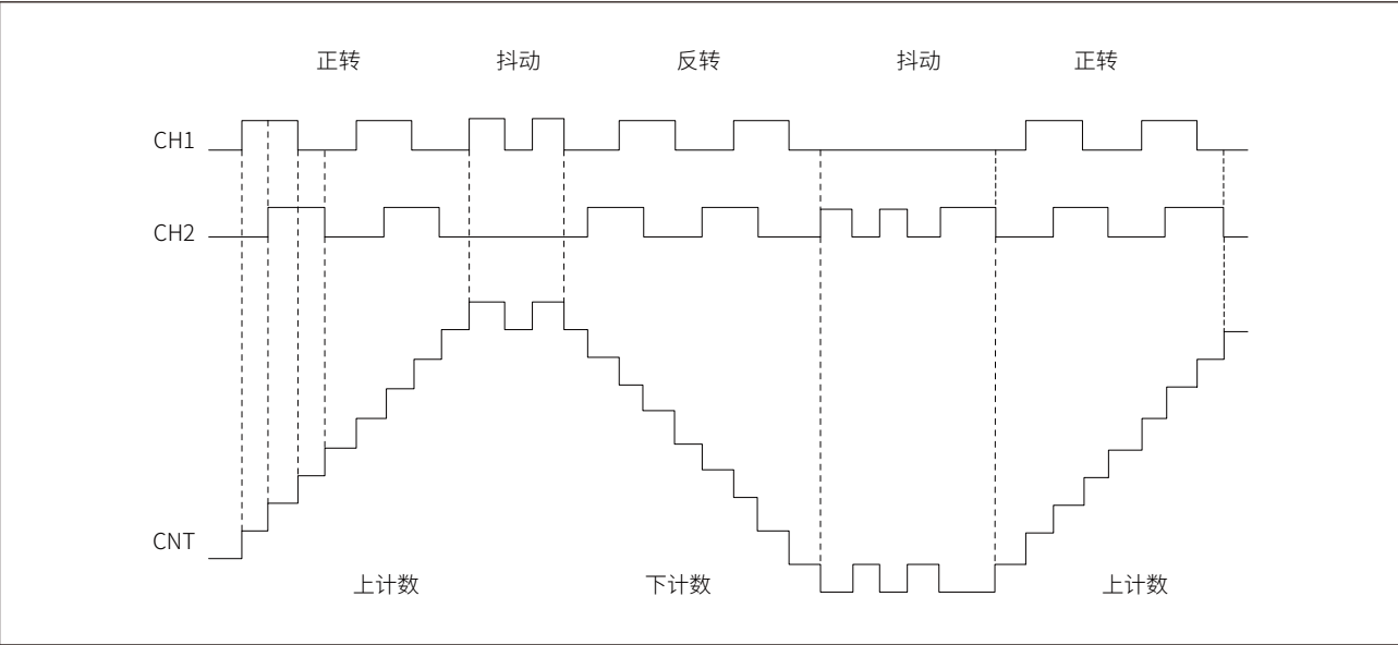
图 17-29 正交编码器模式-x4 模式操作示例
