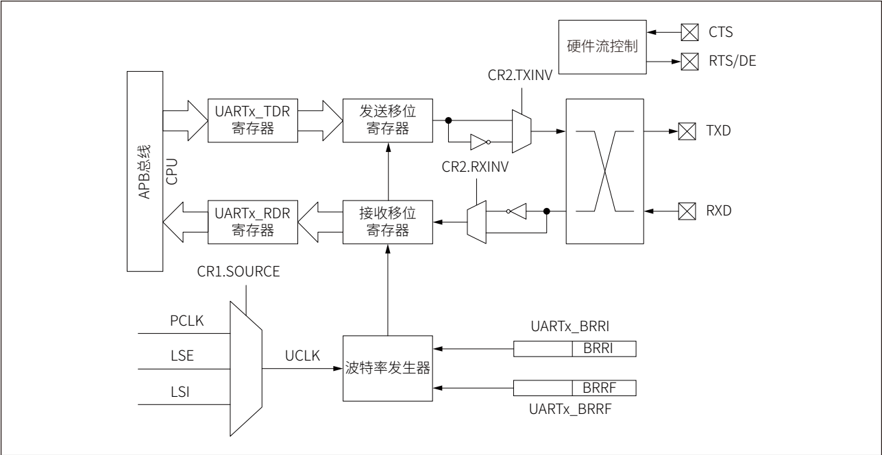
图 21-1 UART 功能框图
