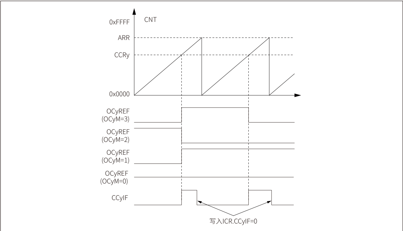
图 16-36 比较匹配输出模式
