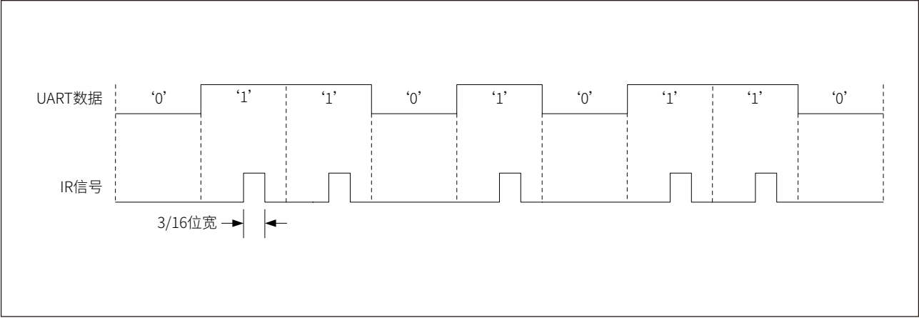
图 24-4 高速 UART 调制方式
