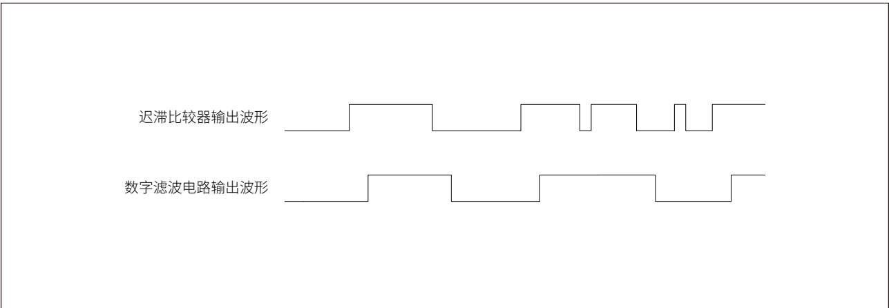
图 28-3 LVD 滤波输出
