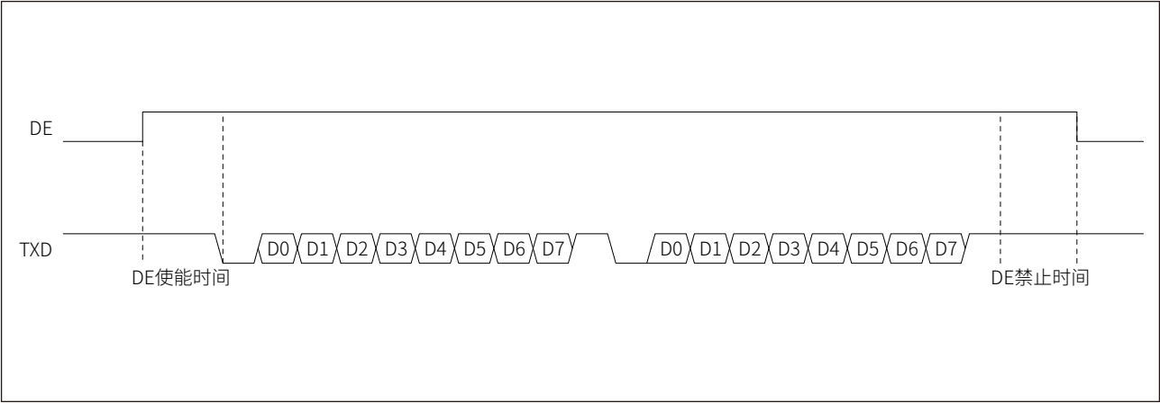
图 21-10 驱动器使能时序
