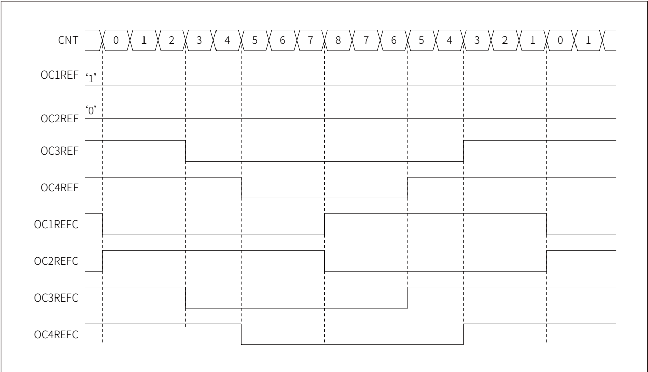
图 16-40 不对称 PWM 模式 1 示例
