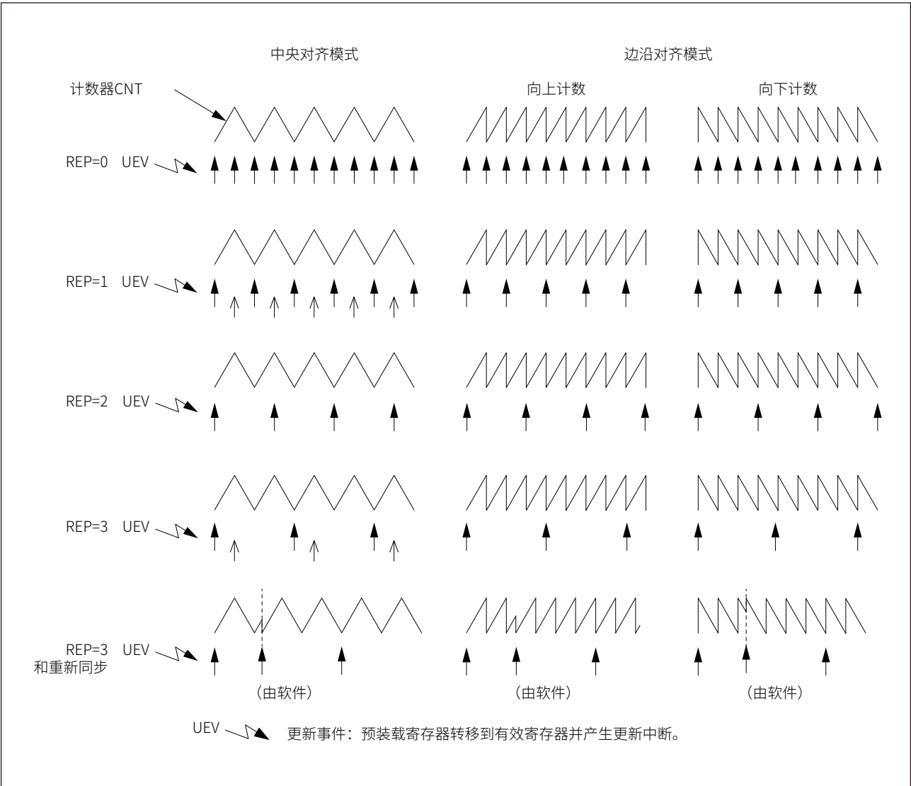
图 17-19 重复计数示例
