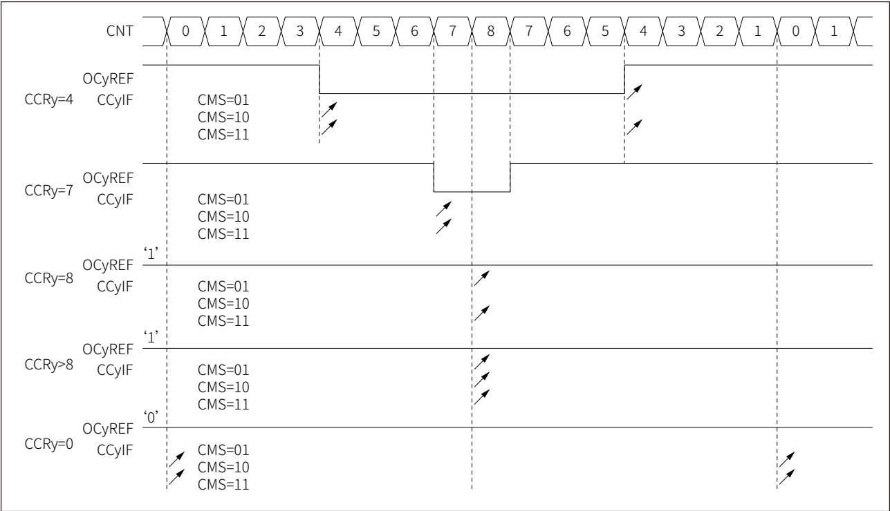
图 17-39 PWM 模式 1，中心对齐模式
