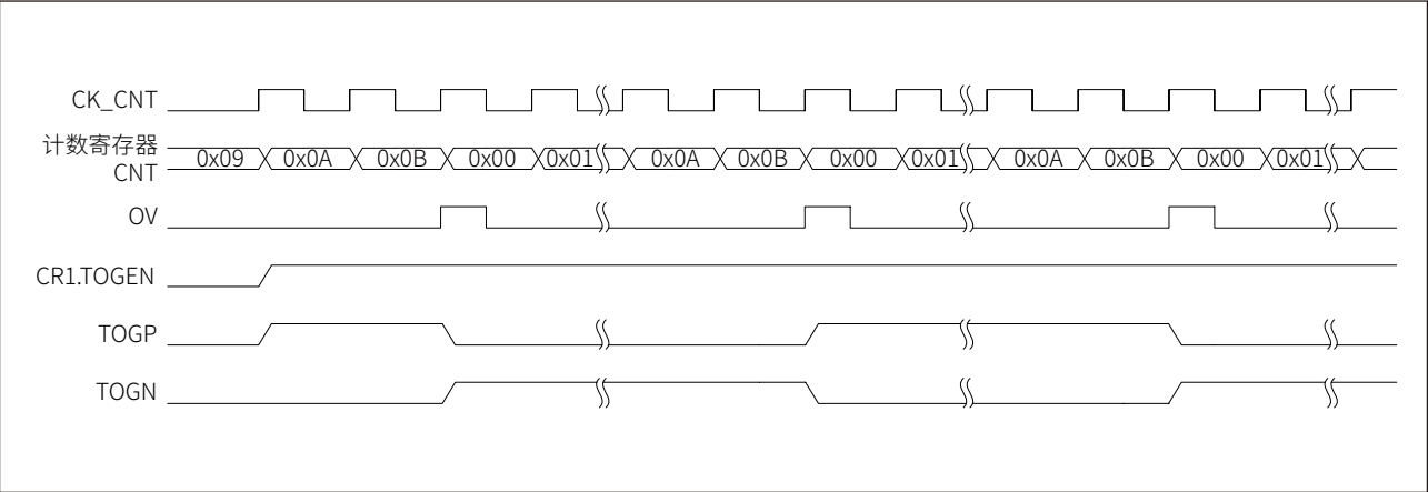
图 14-4 电平翻转输出示意图（ARR=0x0B）
