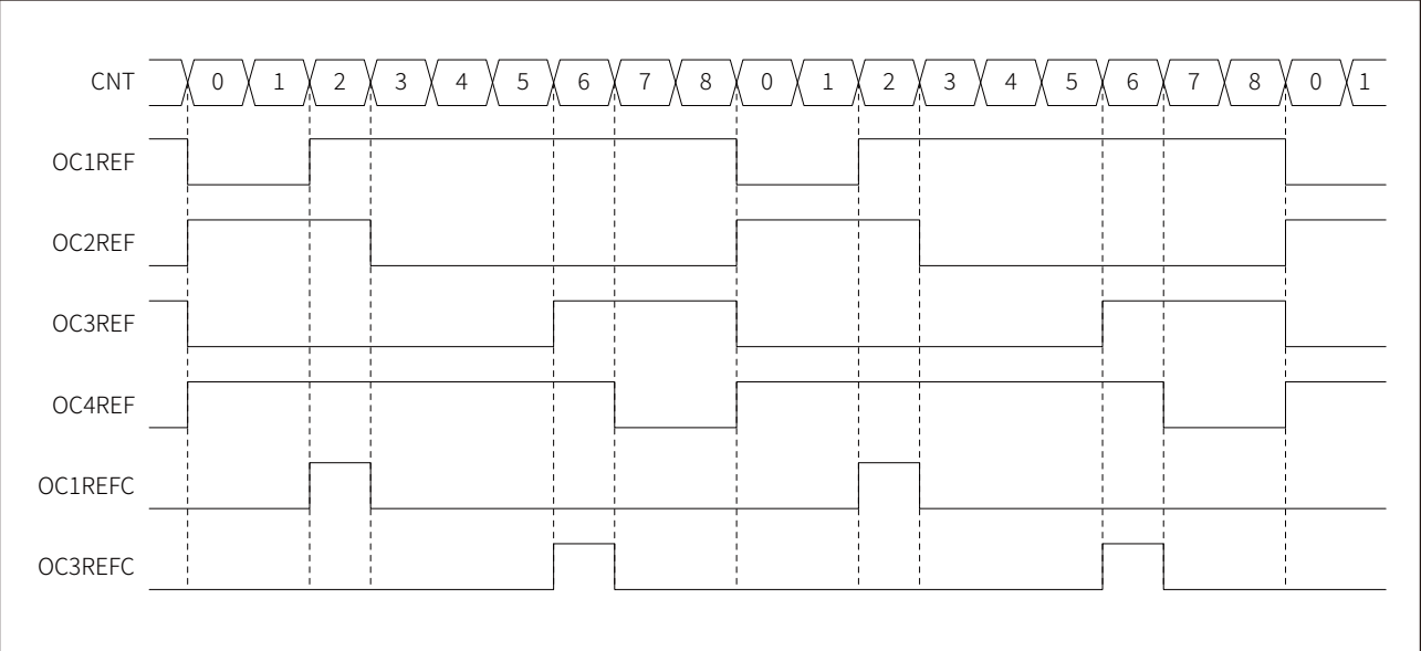
图 16-43 组合 PWM 模式 2 示例
