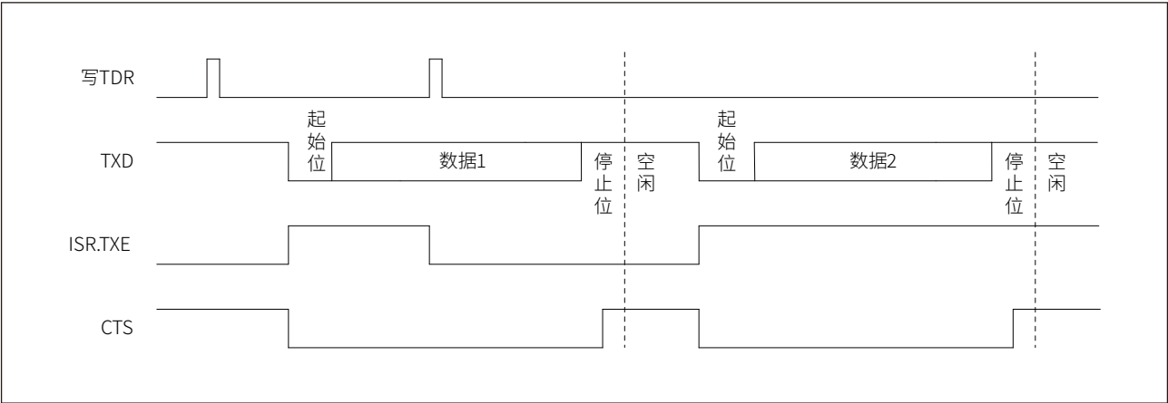
图 21-9 CTS 流控时序
