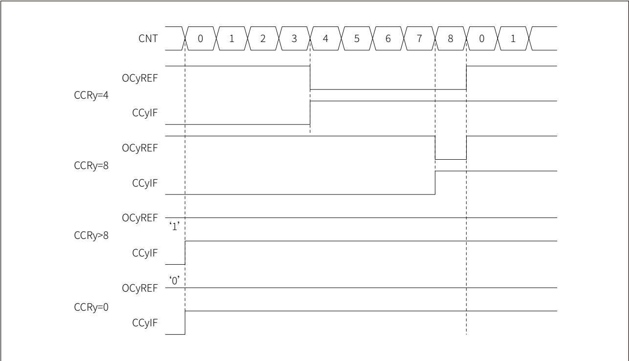
图 17-37 PWM 模式 1，边沿对齐模式，递增计数
