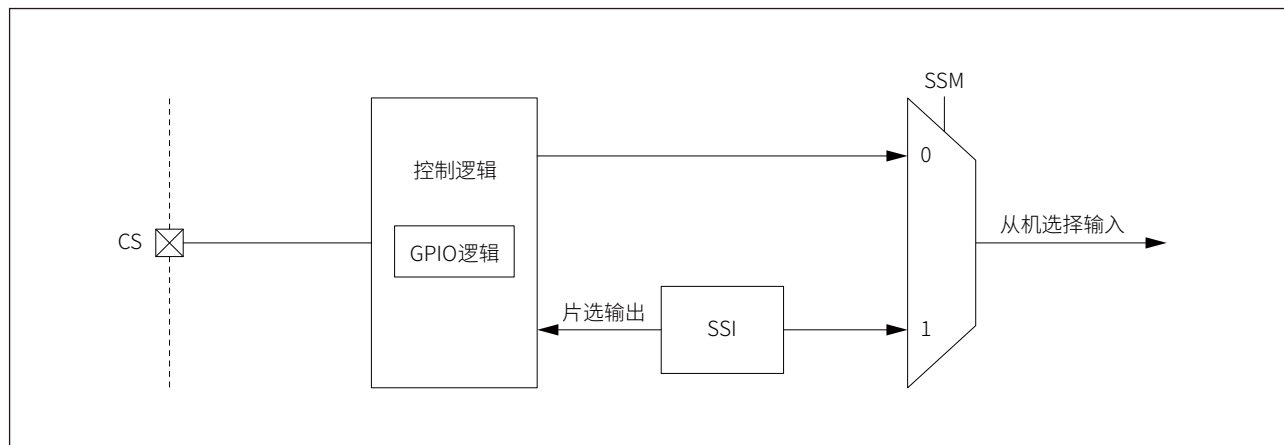
图 22-3 从机选择引脚管理
