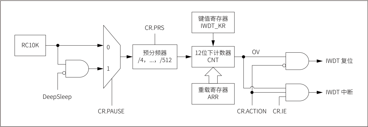
图 19-1 IWDG 功能框图
