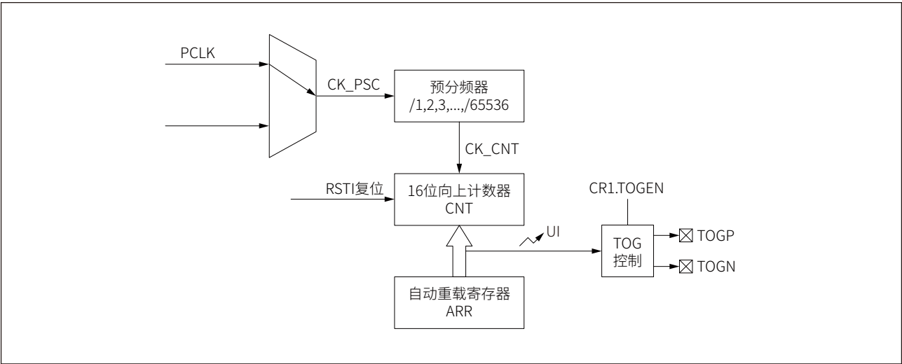
图 14-5 内部计数模式框图
