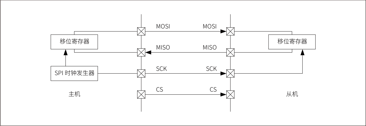
图 22-4 全双工通信模式
