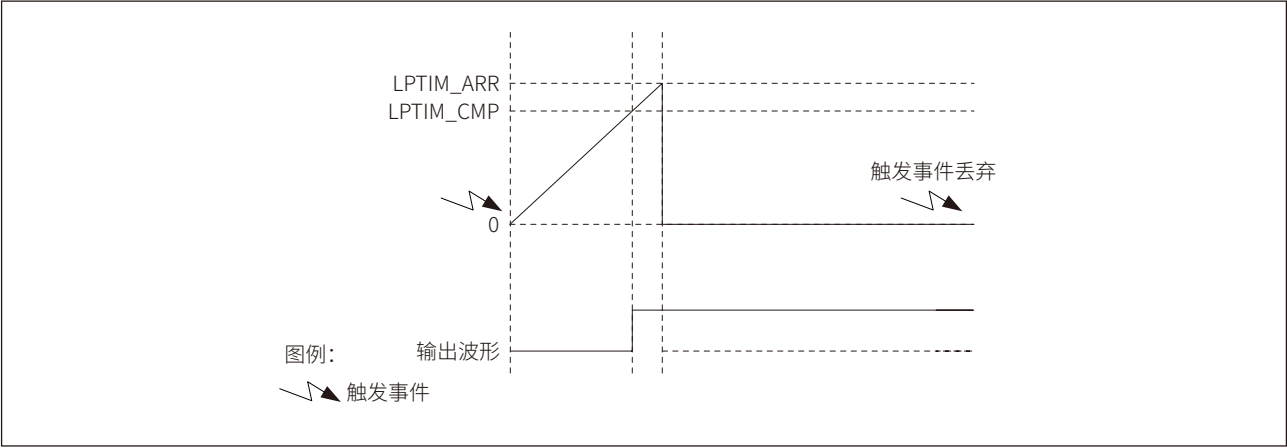
图 15-4 LPTIM 单次置位波形
