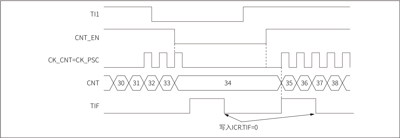
图 16-25 门控模式时序
