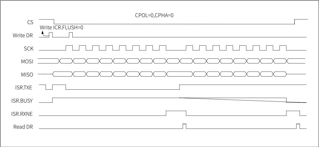
图 22-6 全双工模式下从机收发时序（两个字节）
