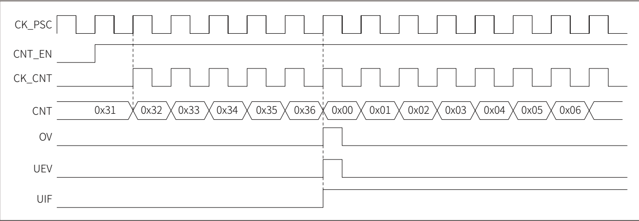
图 17-3 递增计数，内部时钟分频因子为 1
