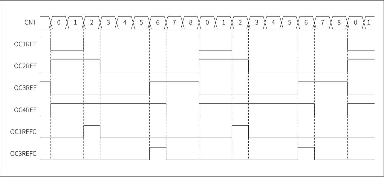
图 17-43 组合 PWM 模式 2 示例
