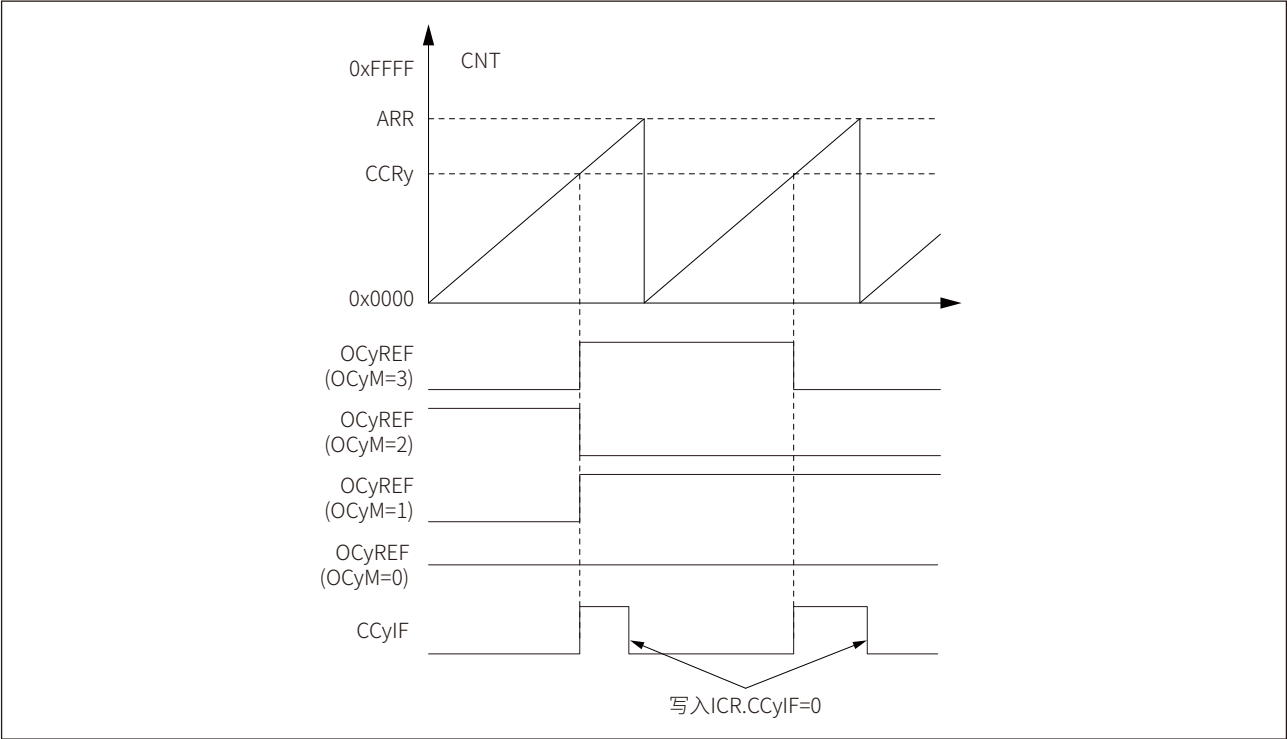
图 17-36 比较匹配输出模式
