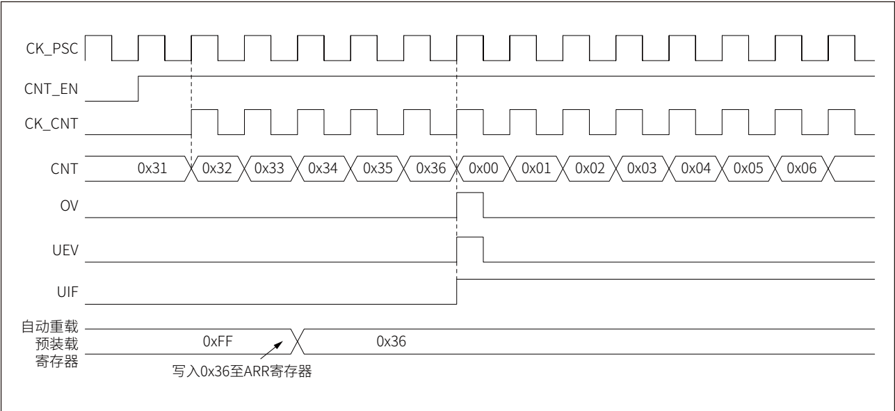
图 16-8 递增计数，当重载缓存使能时的更新事件 (GTIMx_CR1.ARPE=1)
