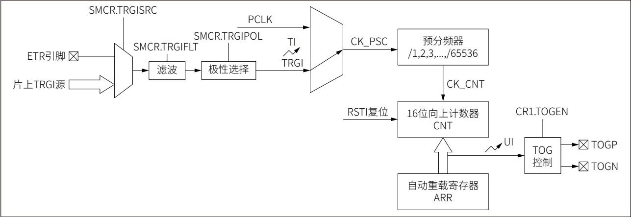
图 14-6 外部计数模式框图
