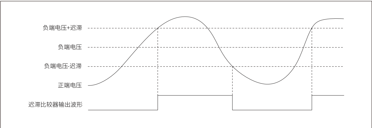
图 27-3 VC 迟滞功能
