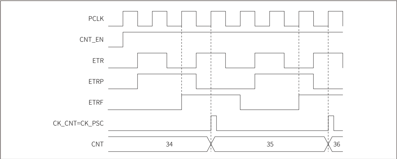
图 16-23 外部时钟模式 2 时序示例
