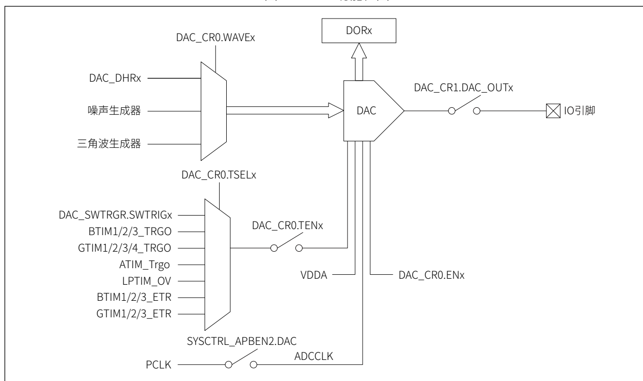
图 26-1 DAC功能框图
