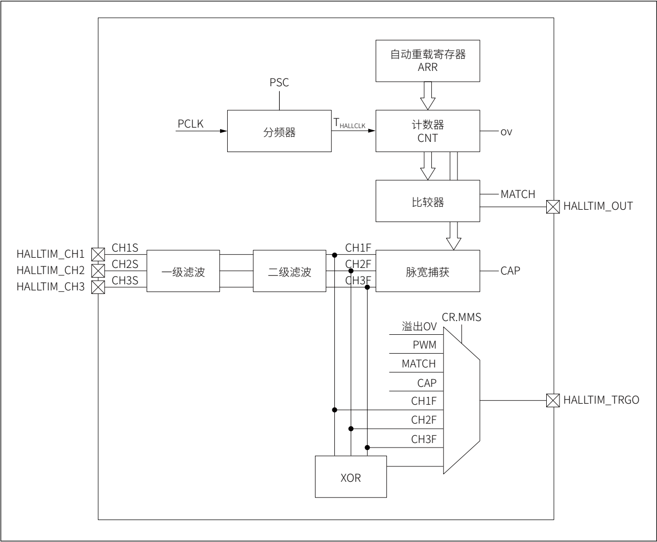
图 18-1 HALLTIM 功能框图
