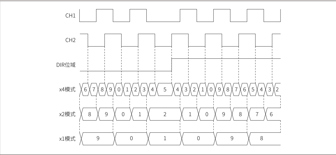
图 17-30 各正交编码器模式计数示例
