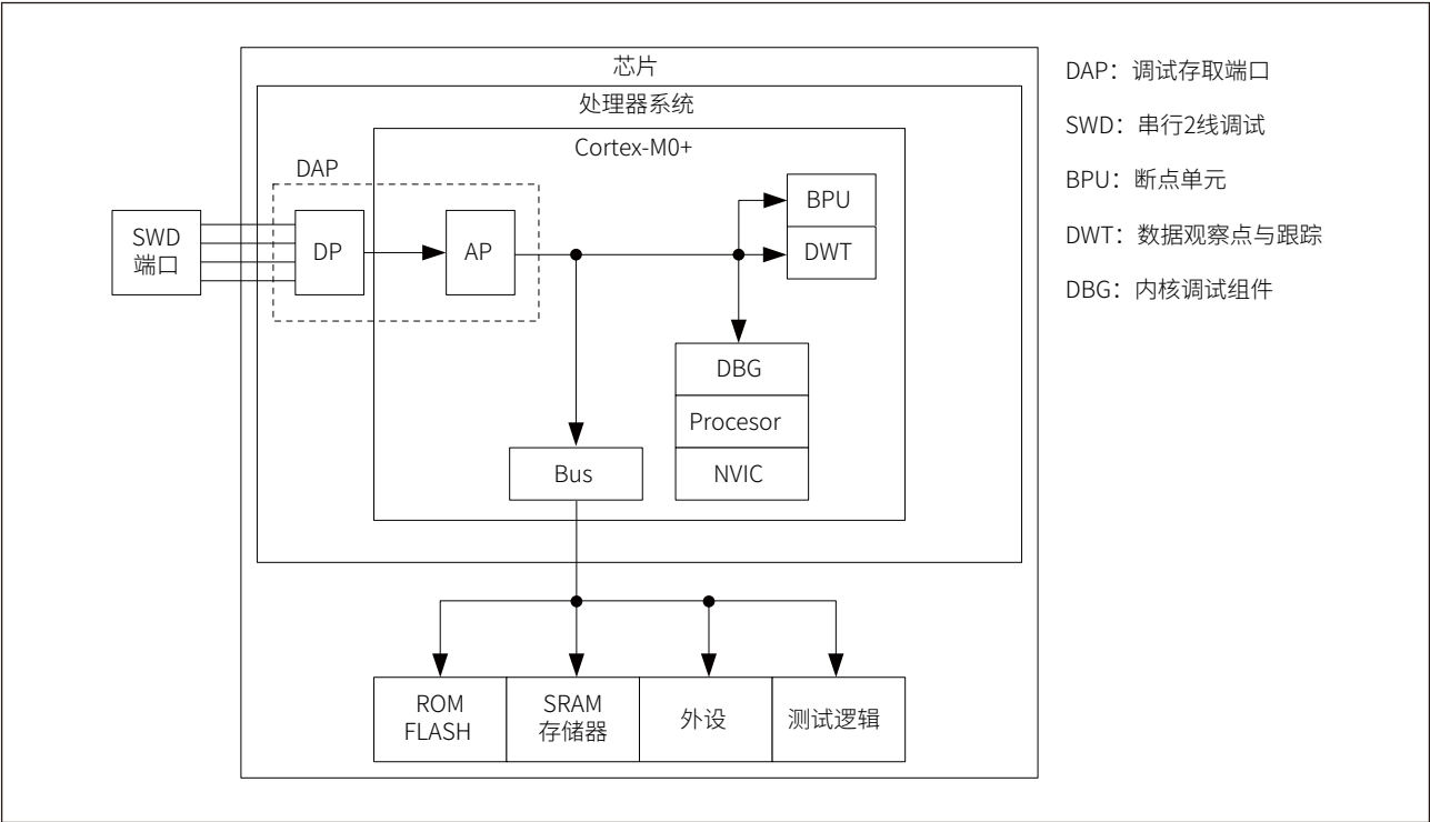
图 30-1 SWD 功能框图
