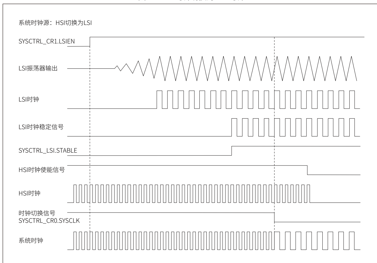
图 4-6 HSI 时钟切换为 LSI 时钟
