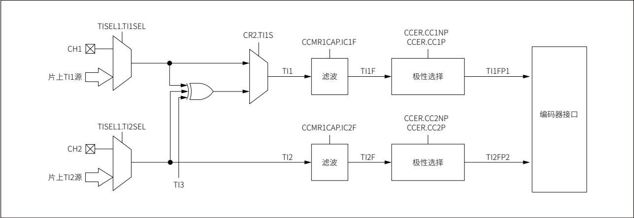
图 17-28 编码器模式框图
