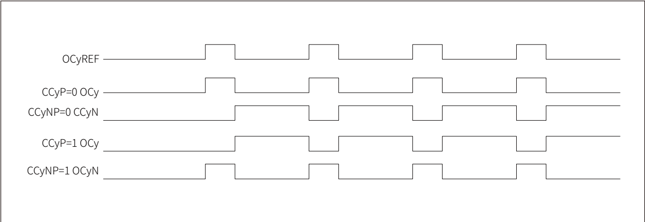
图 17-46 互补 PWM 输出波形
