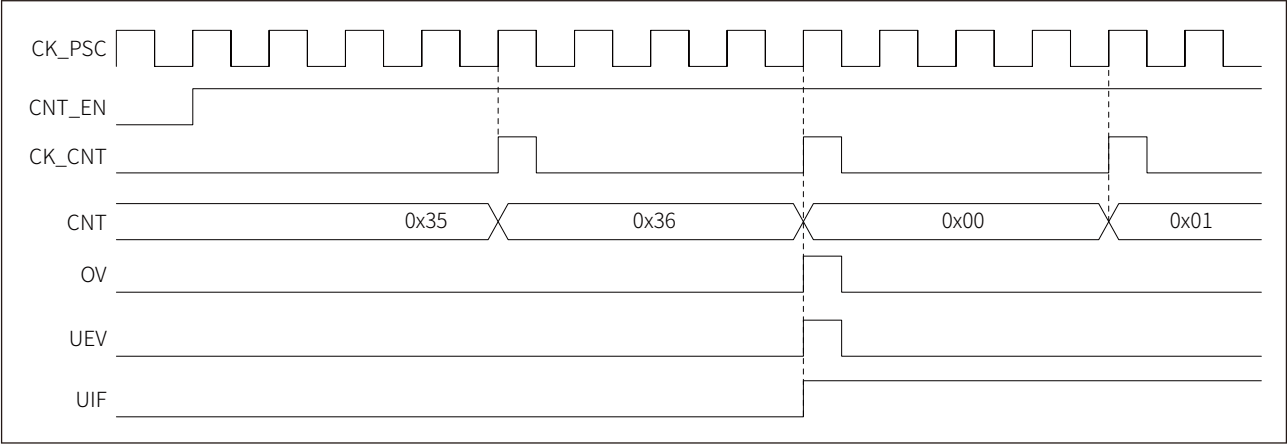
图 16-6 递增计数，内部时钟分频因子为 N
