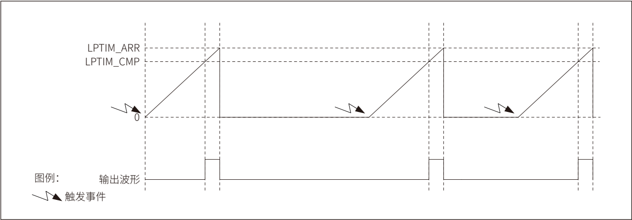
图 15-3 LPTIM 单次模式
