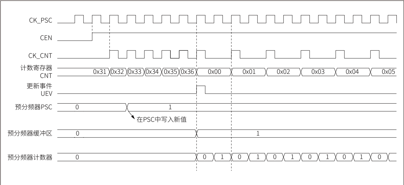
图 16-2 预分频器分频由 1 变为 2 时的时序图
