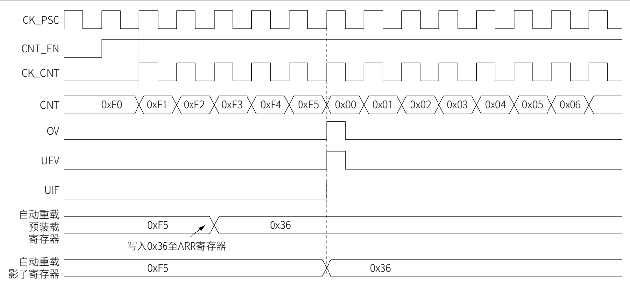
图 17-8 递增计数，当重载缓存使能时的更新事件 (ATIM_CR1.ARPE=1)
