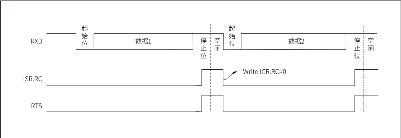
图 21-8 RTS 流控时序
