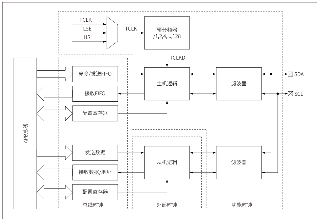
图 23-6 I2C 功能框图
