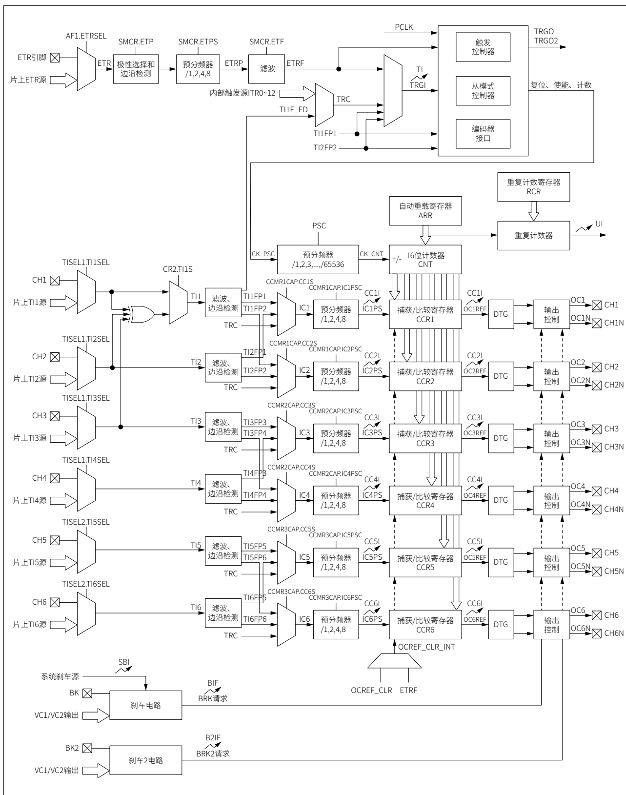
图 17-1 ATIM 功能框图
