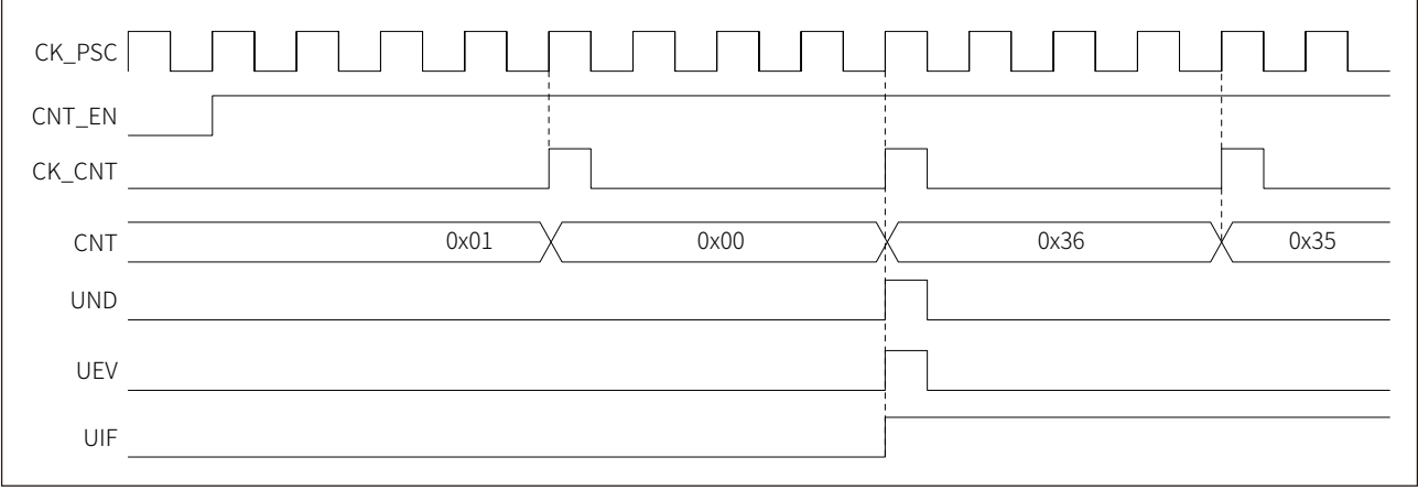
图 17-11 递减计数，内部时钟分频因子为 4
