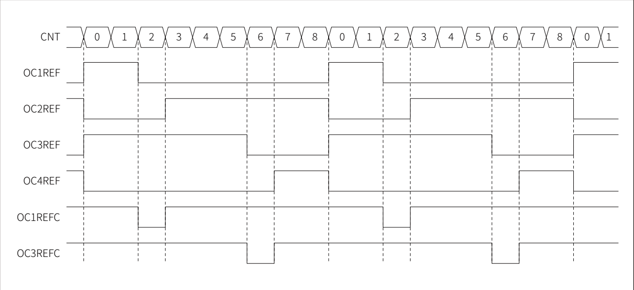
图 16-42 组合 PWM 模式 1 示例
