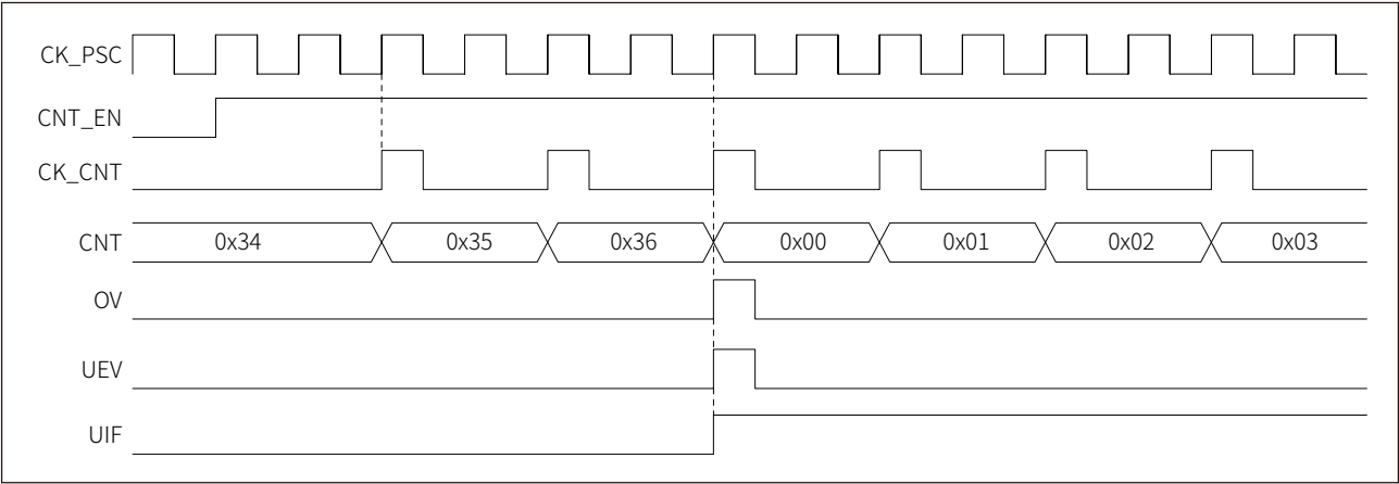
图 16-5 递增计数，内部时钟分频因子为 4
