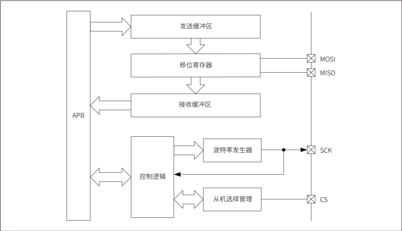
图 22-1 SPI 功能框图
