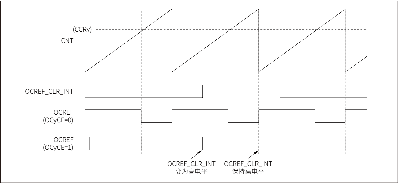
图 17-53 OCyREF 清零示例
