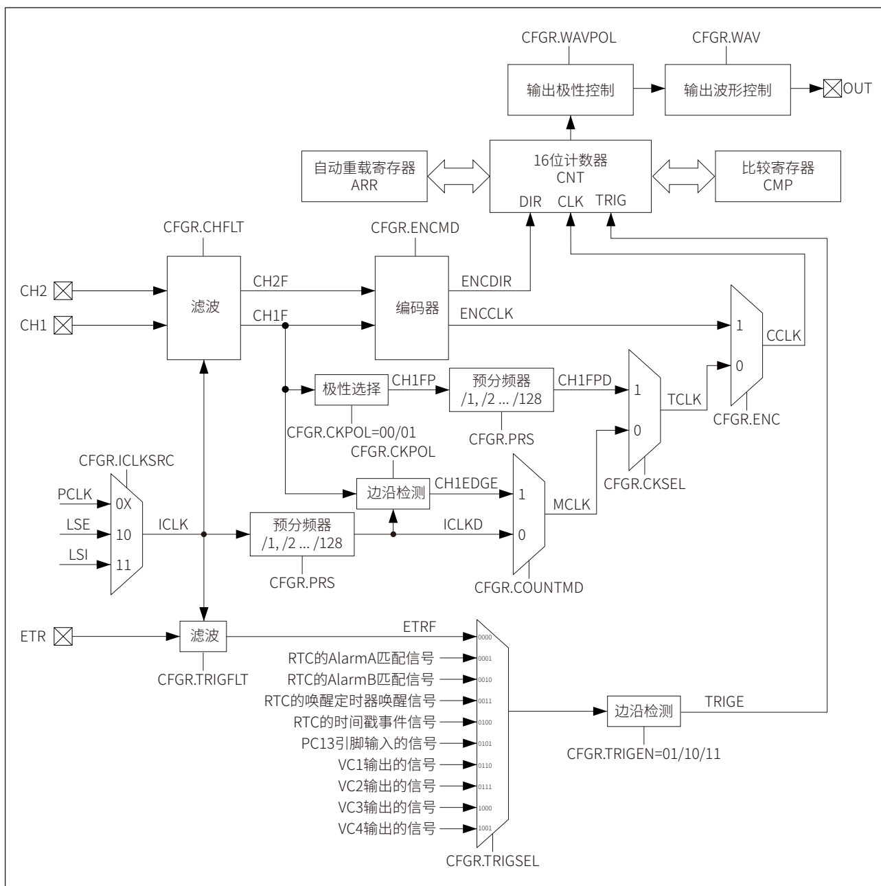
图 15-1 LPTIM功能框图
