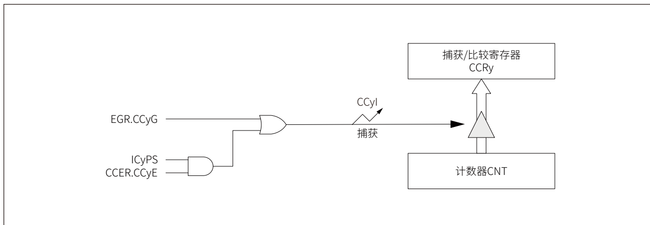
图 17-34 输入捕获模式框图
