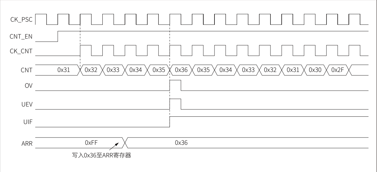
图 17-18 中心对齐模式，当重载缓存使能时的更新事件 (ATIM_CR1.ARPE=1)
