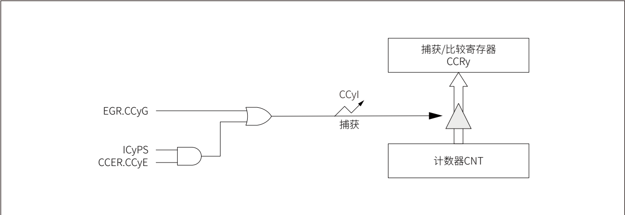
图 16-33 输入捕获模式框图
