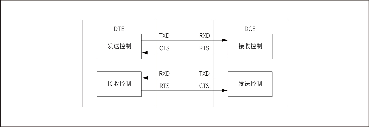
图 21-7 硬件流控示意图
