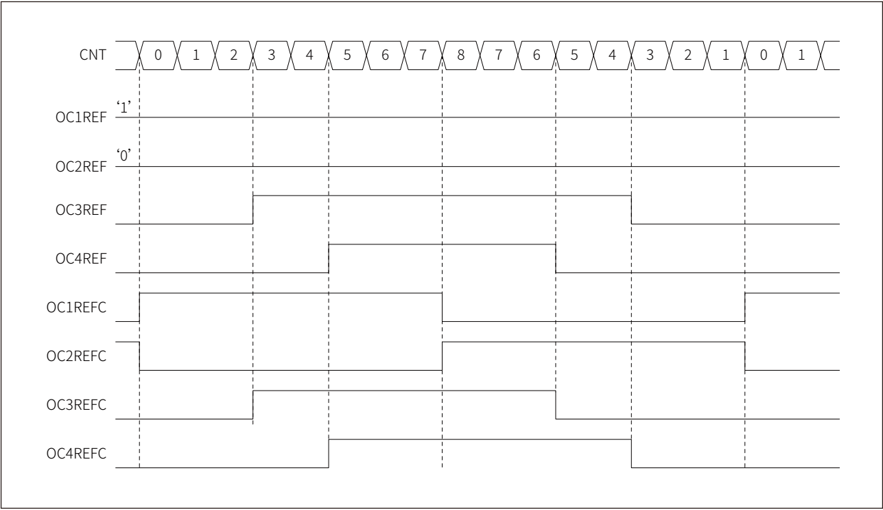
图 16-41 不对称 PWM 模式 2 示例
