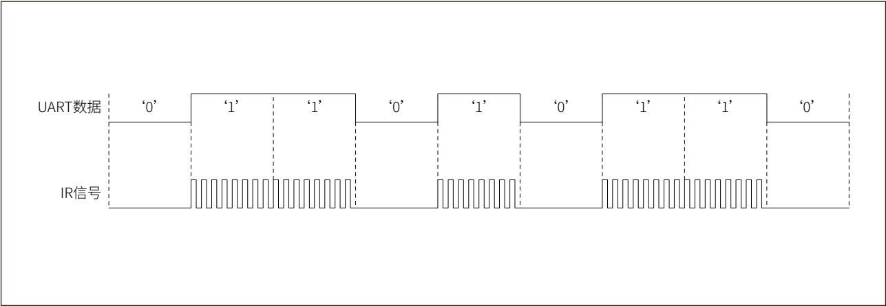
图 24-3 UART 调制方式
