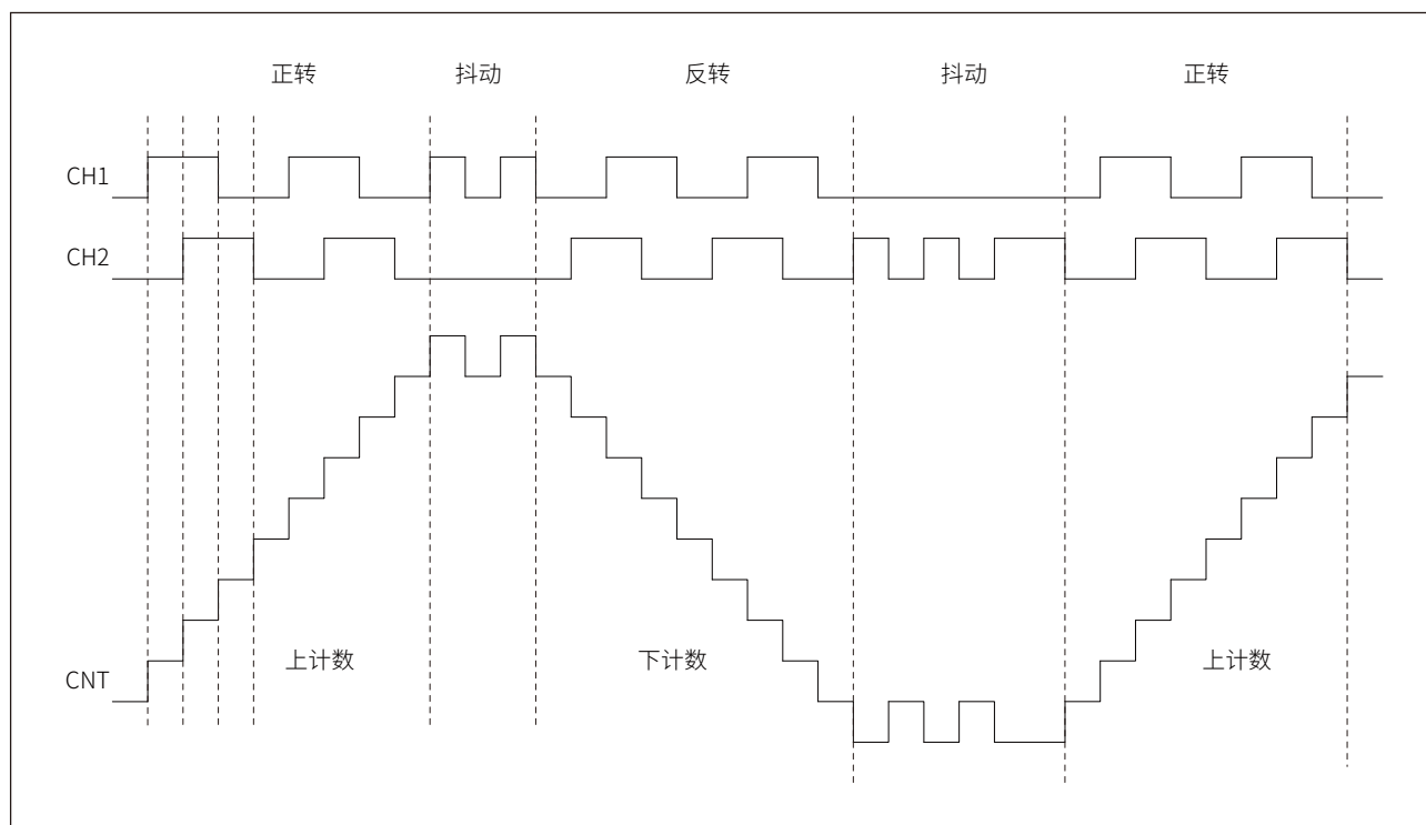
图 15-7 编码器模式计数示例
