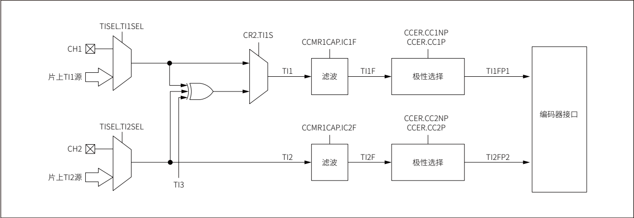
图 16-27 编码器模式框图
