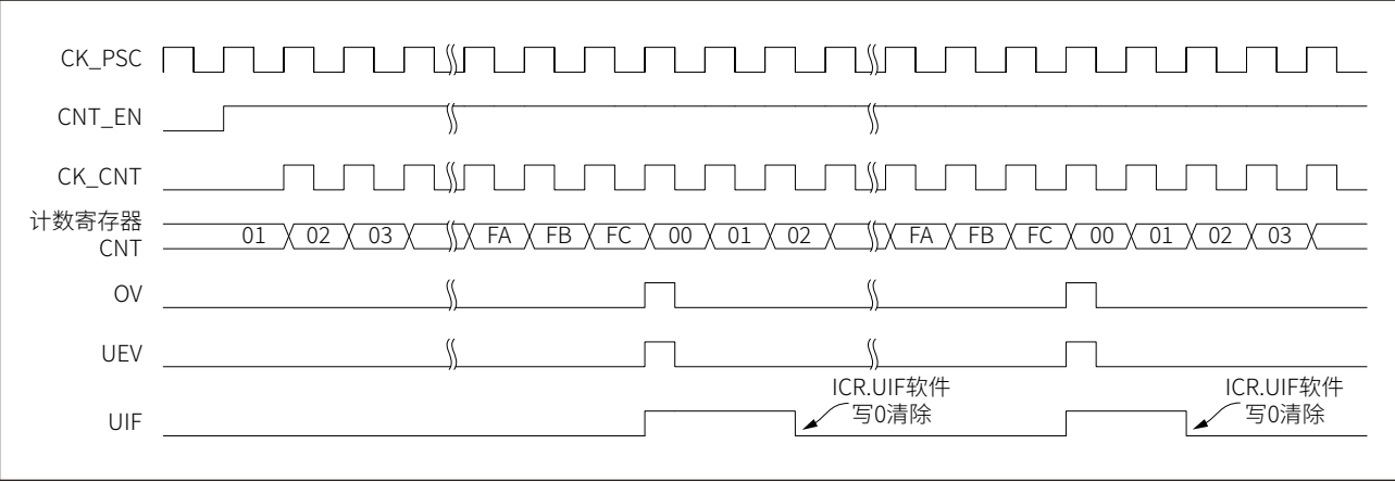
图 14-3 连续计数模式示例
