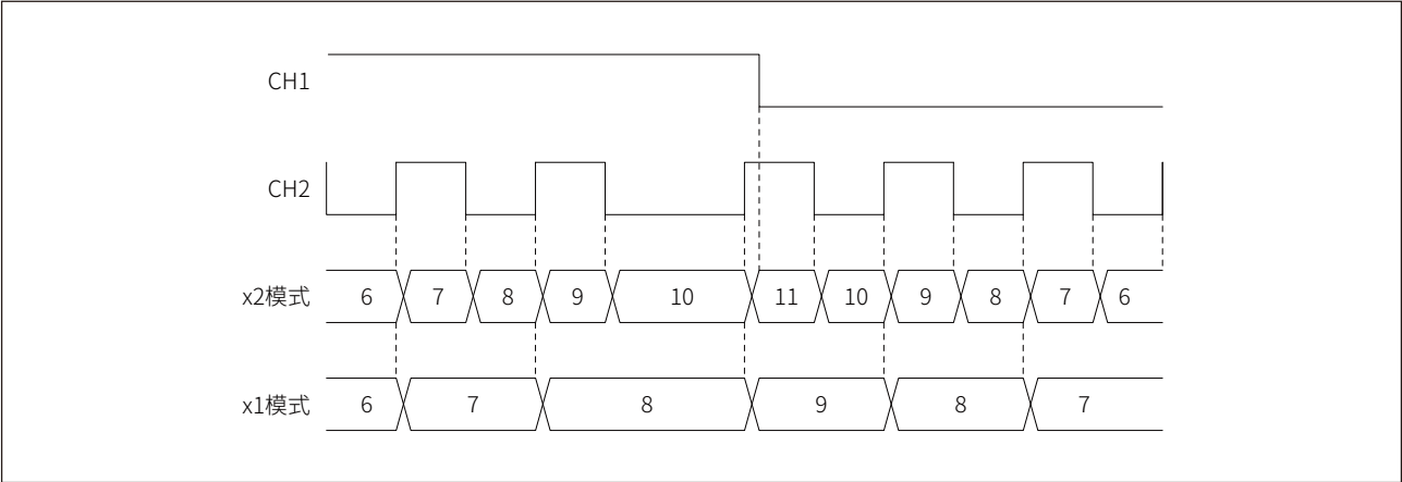
图 16-30 时钟加方向编码器模式计数示例
