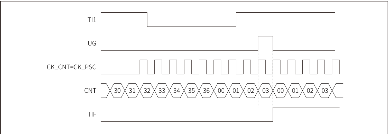
图 16-24 复位模式时序
