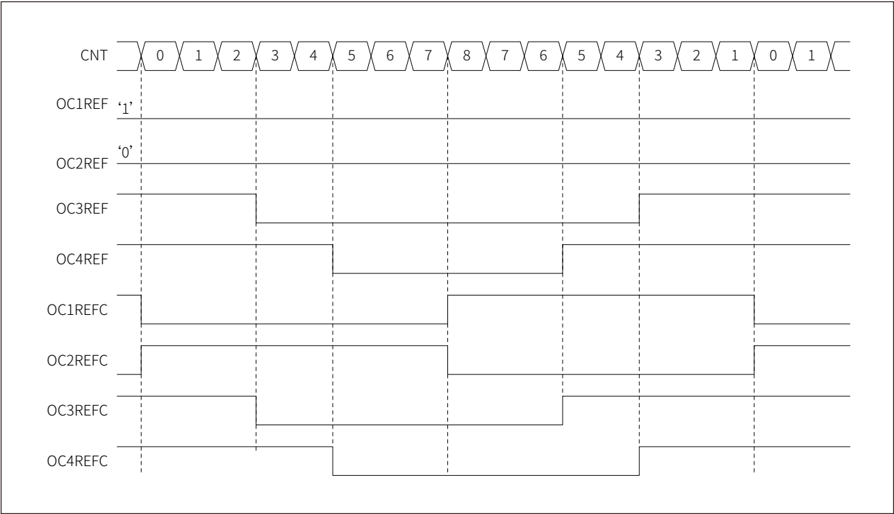
图 17-40 不对称 PWM 模式 1 示例
