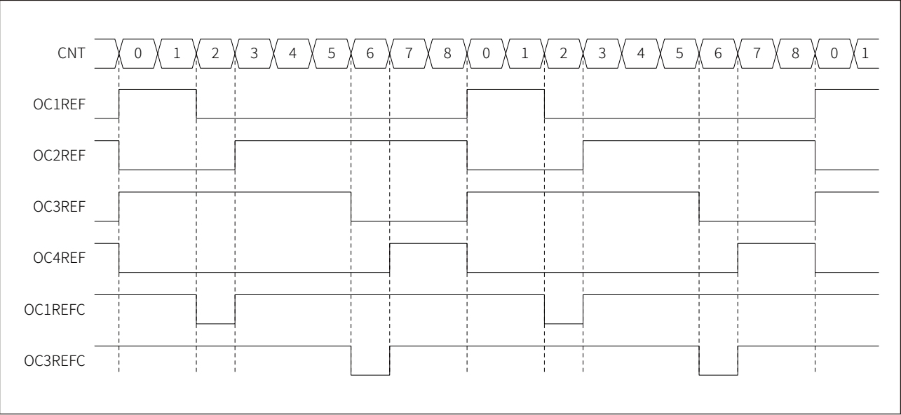
图 17-42 组合 PWM 模式 1 示例
