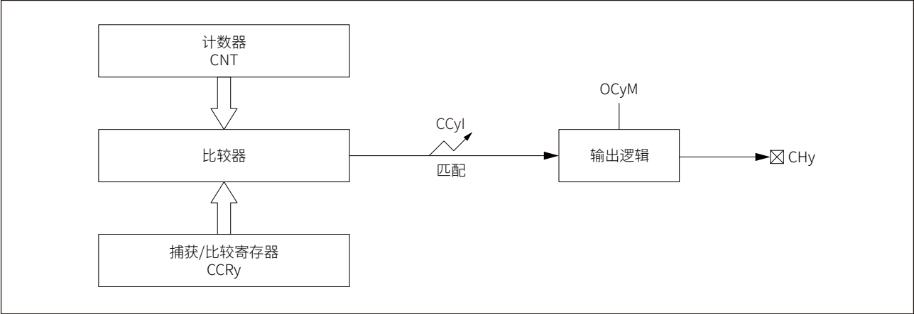
图 16-35 输出比较模式框图
