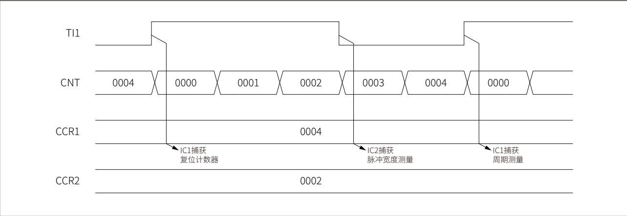
图 16-34 PWM 输入模式时序
