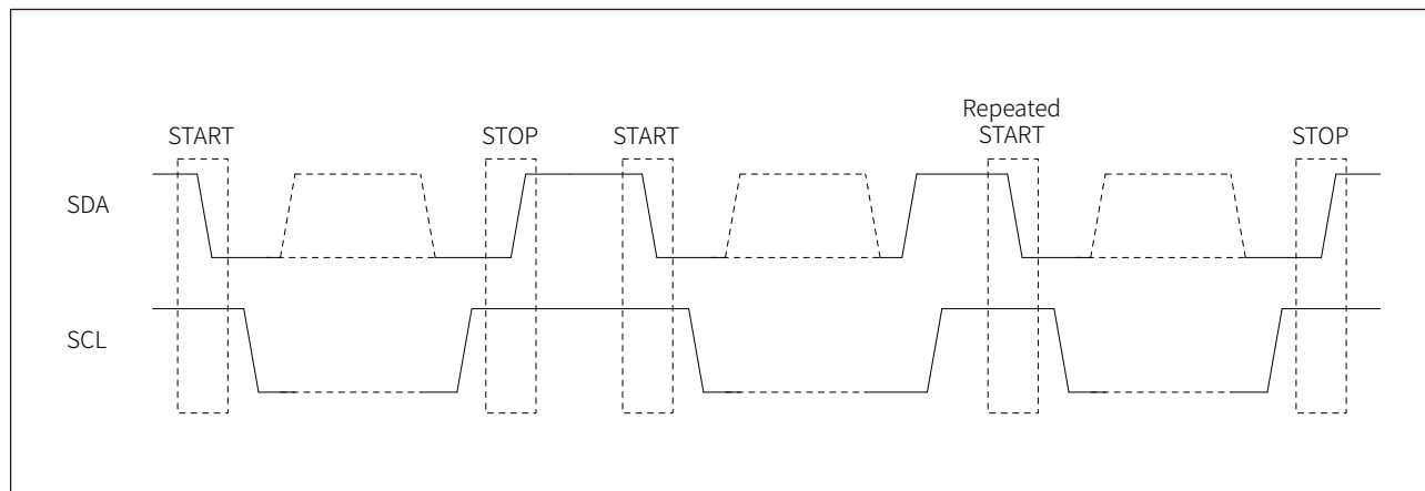
图 23-2 起始和停止信号
