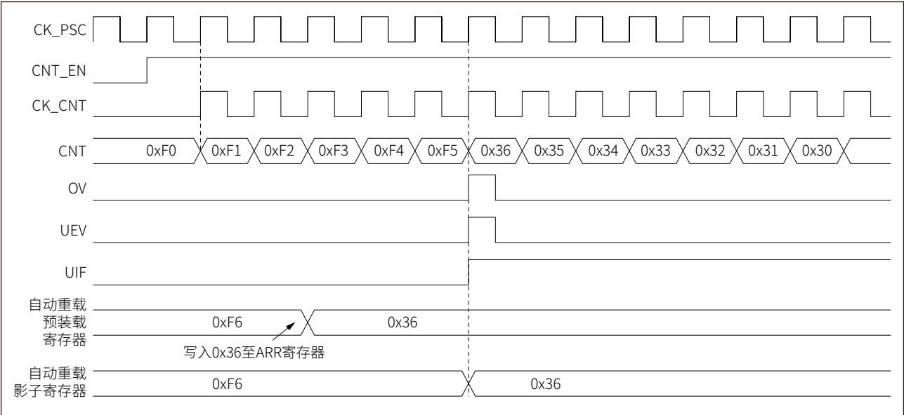
图 16-18 中心对齐模式，当重载缓存使能时的更新事件 (GTIMx_CR1.ARPE=1)
