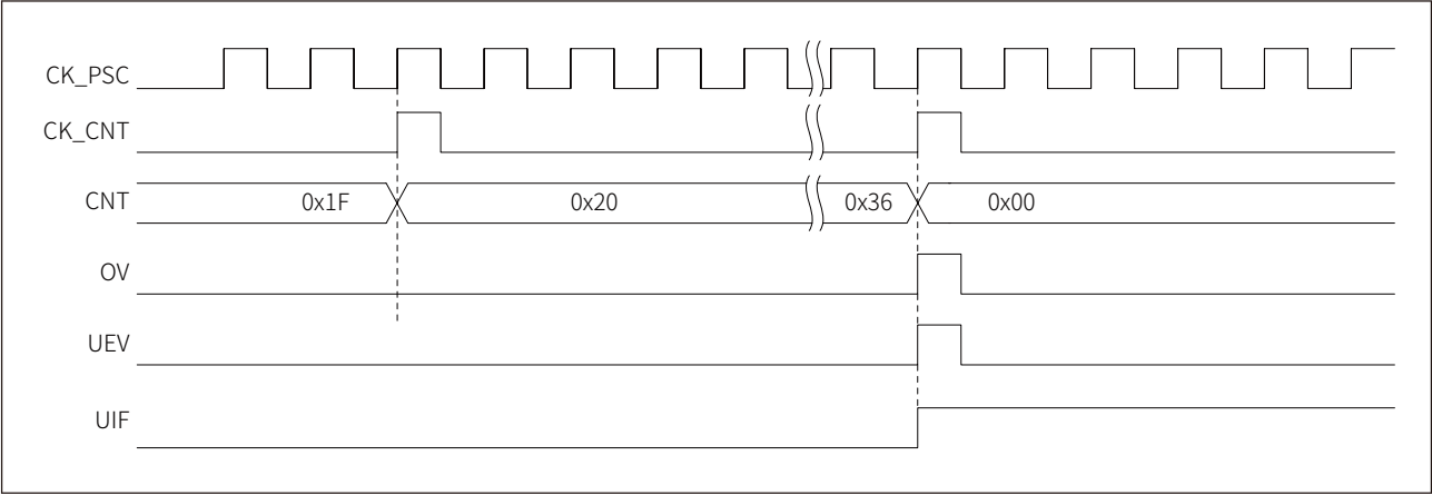
图 16-6 递增计数，内部时钟分频因子为 N
