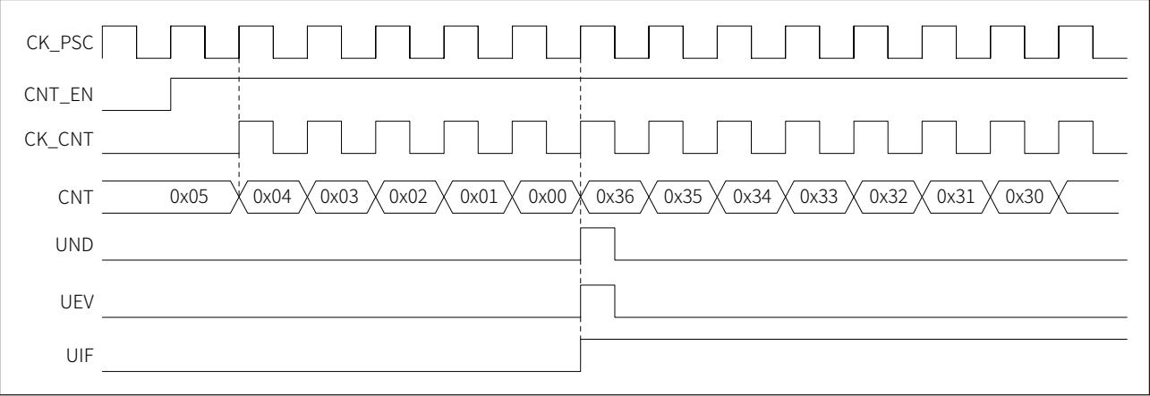
图 16-10 递减计数，内部时钟分频因子为 2
