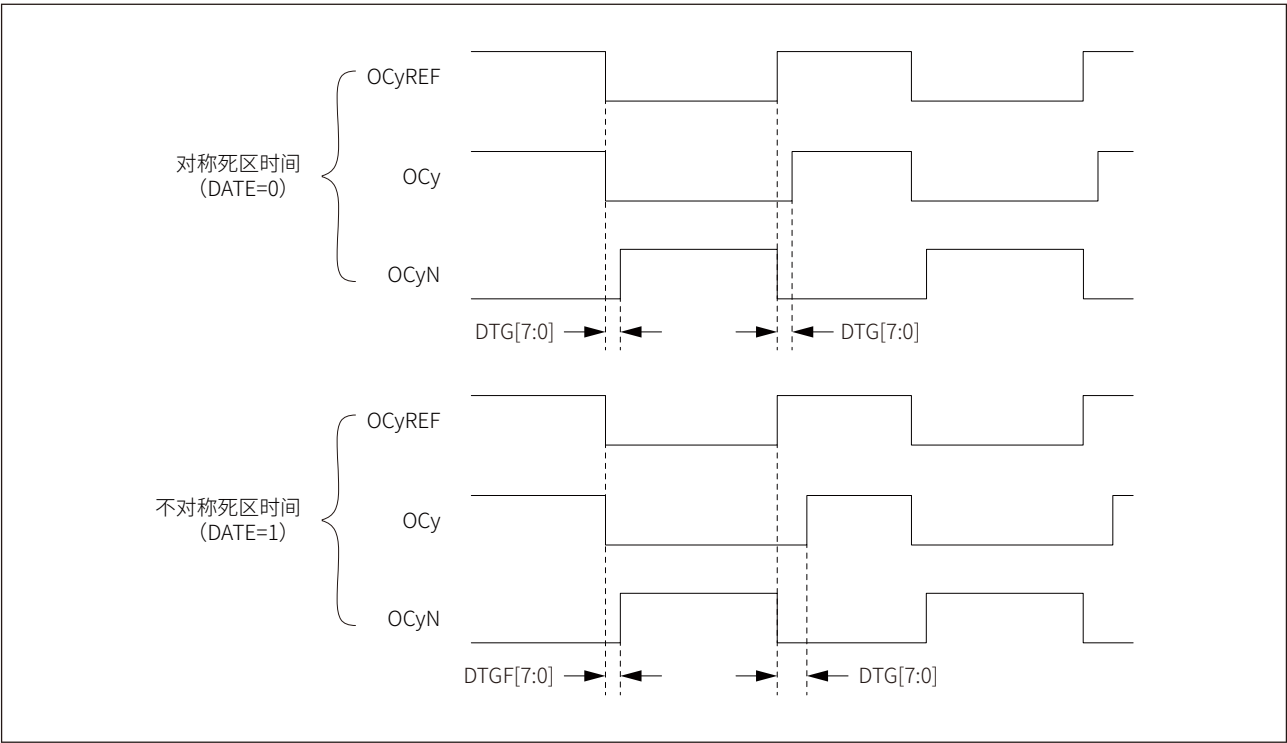
图 17-47 带死区插入的互补 PWM 输出波形
