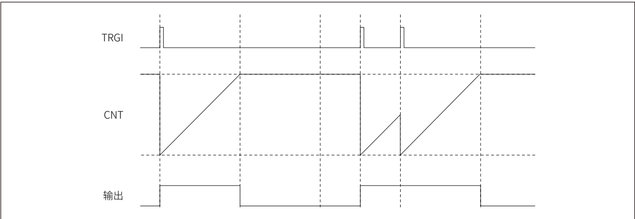
图 17-52 可再触发单脉冲模式 2 示例
