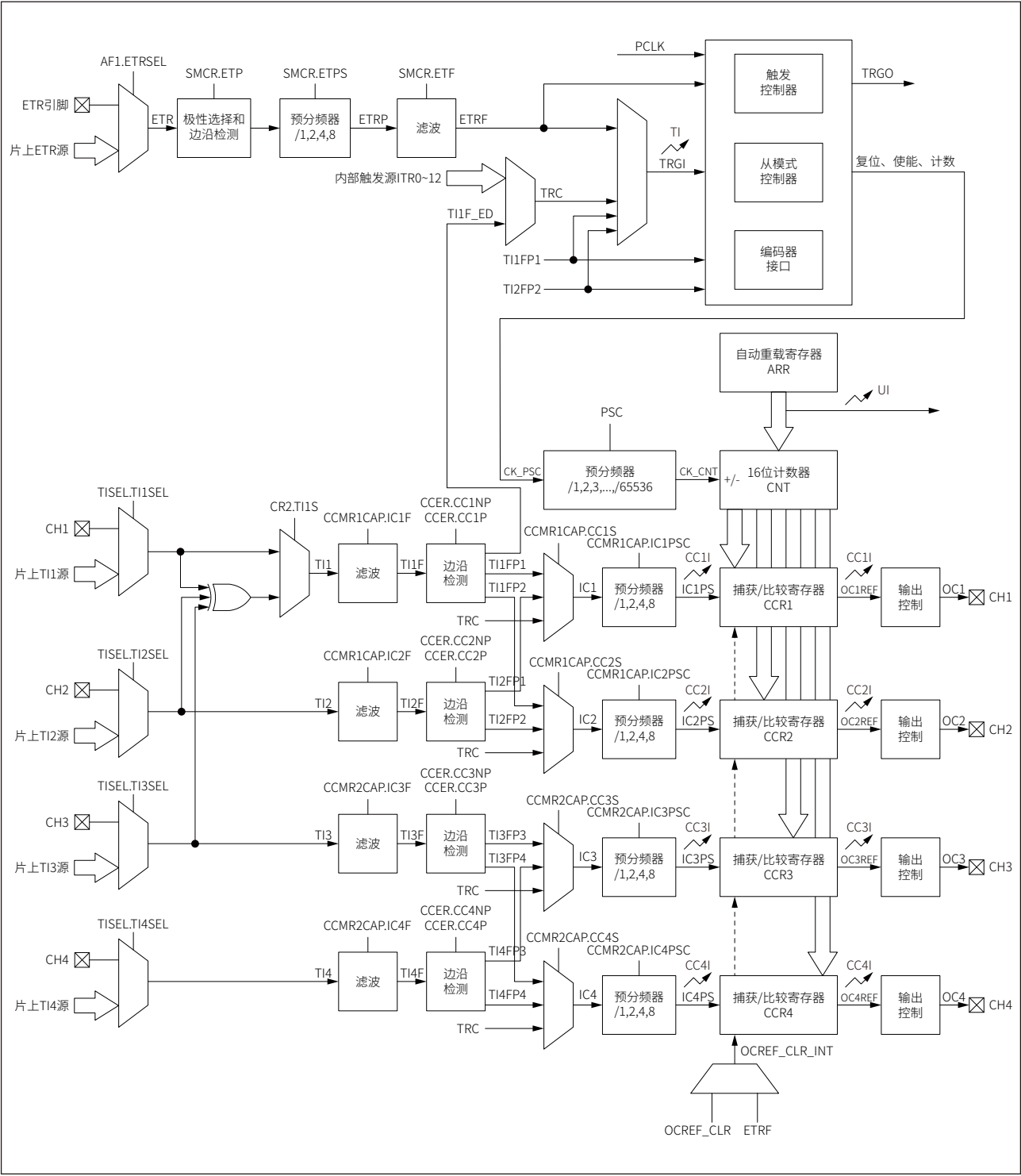
图 16-1 GTIM 功能框图
