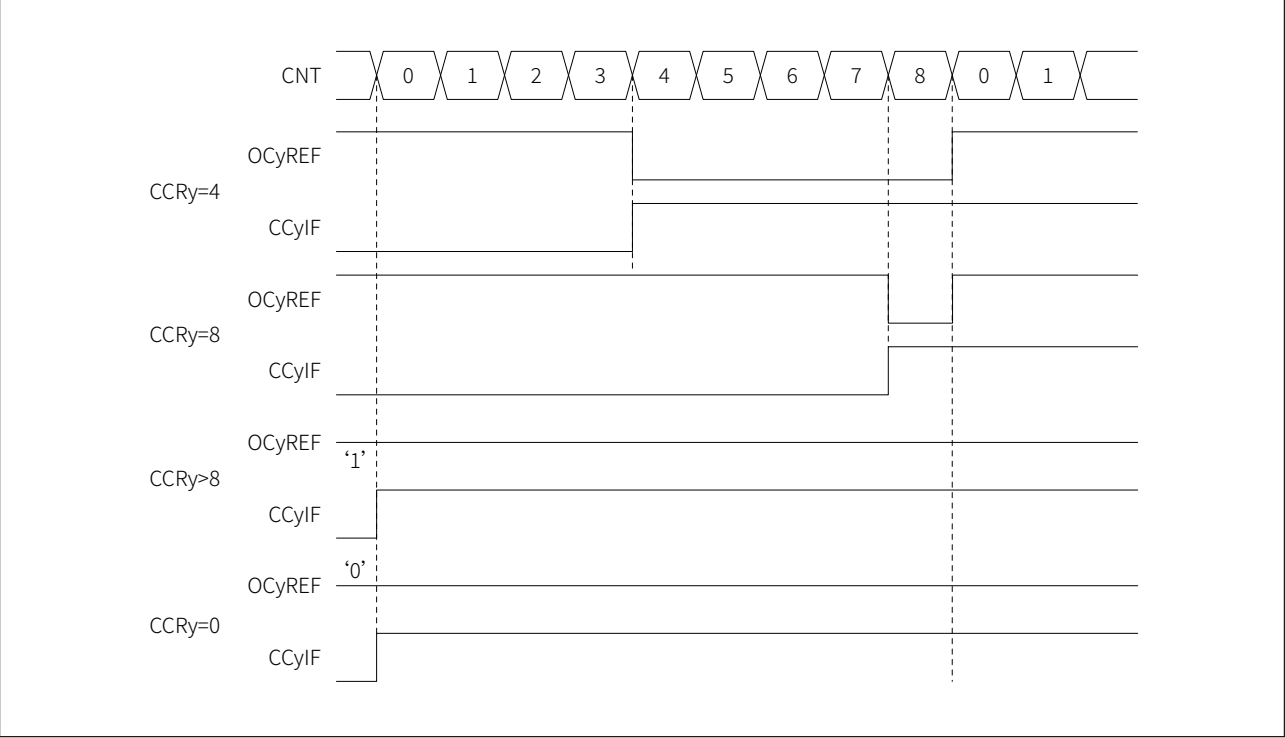
图 16-37 PWM 模式 1，边沿对齐模式，递增计数
