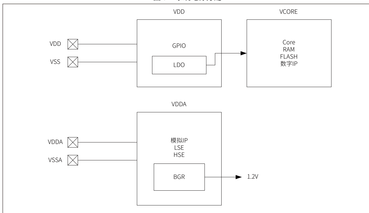
图 3-1 系统电源分配
