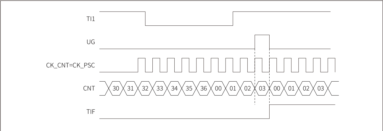
图 17-25 复位模式时序
