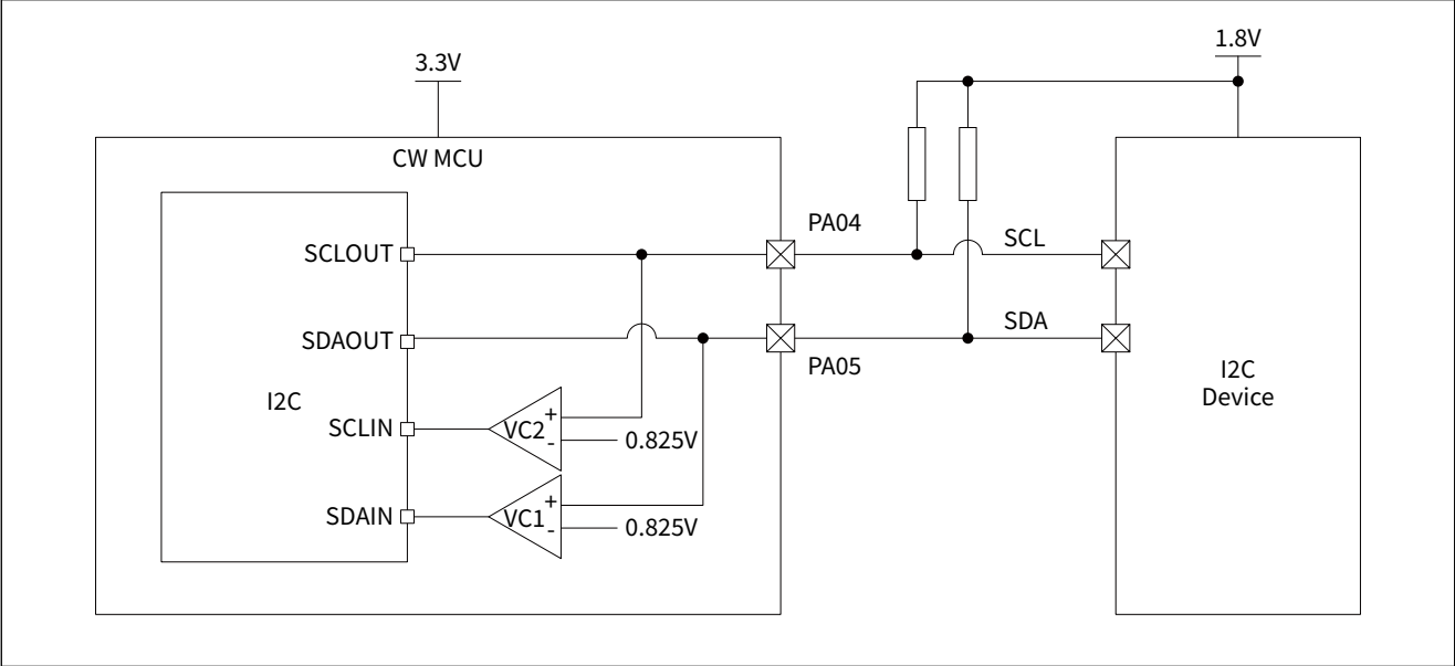
图 18-7 不同电压器件通信示意图
