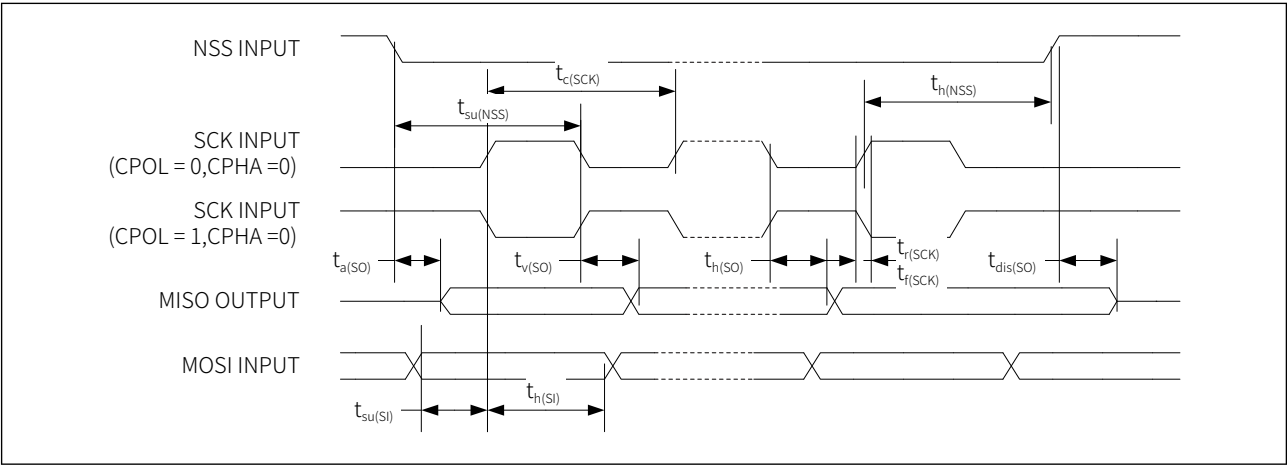
图 7-11 SPI 时序图-从模式 CPHA=0
