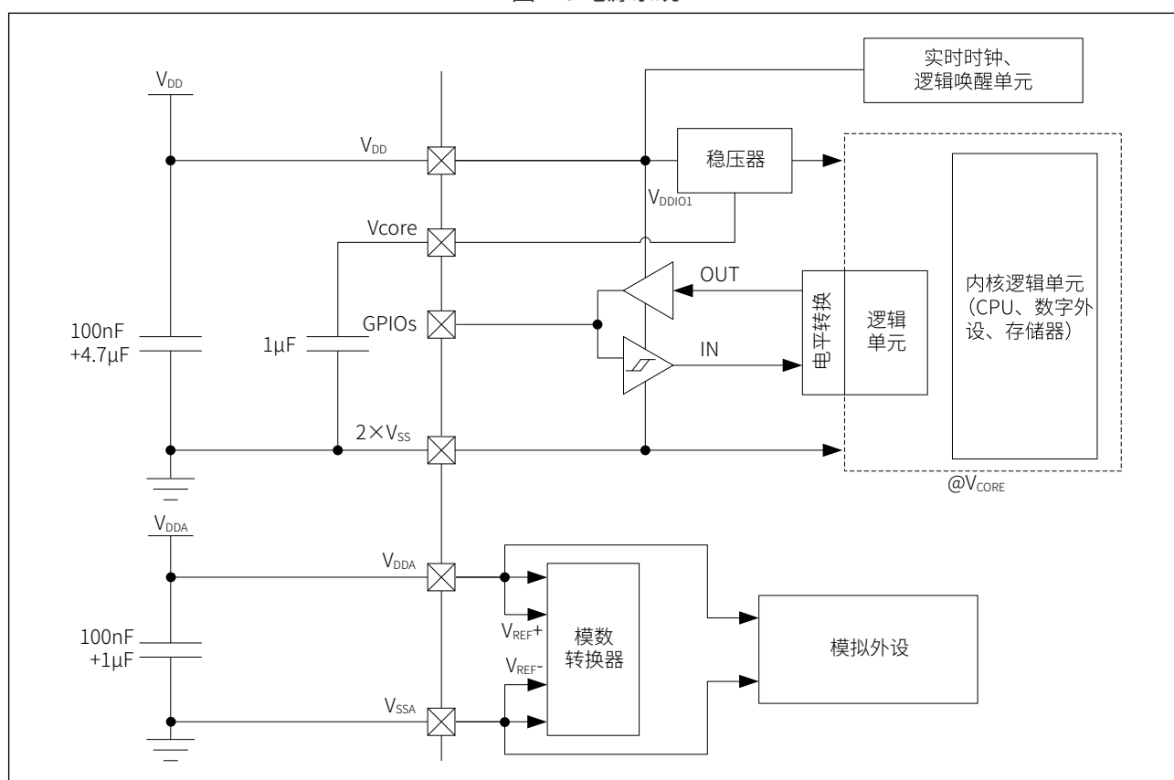
图 7-3 电源系统
