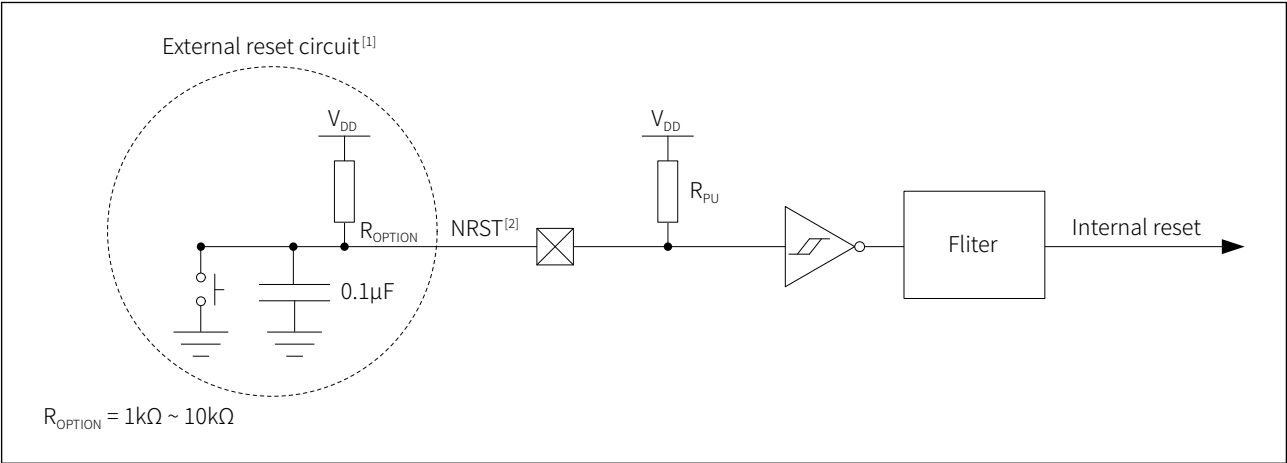
图 7-8 推荐的 NRST 引脚电路
