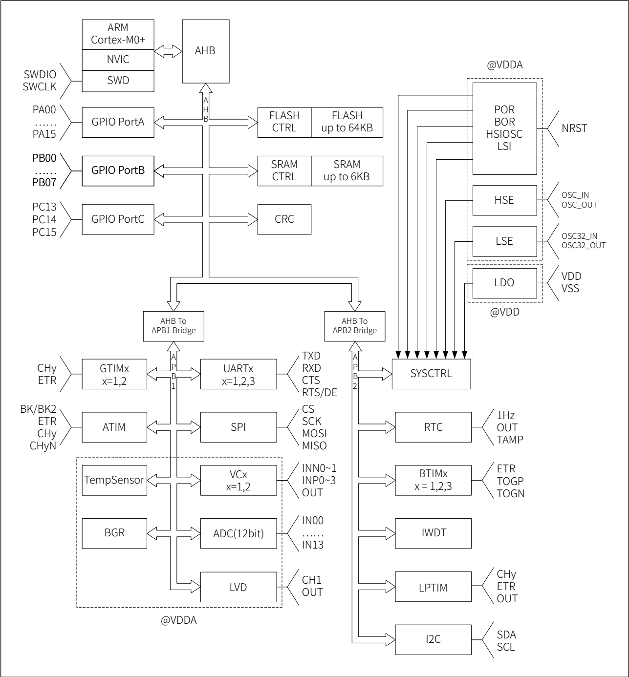
图 3-1 内部框图
