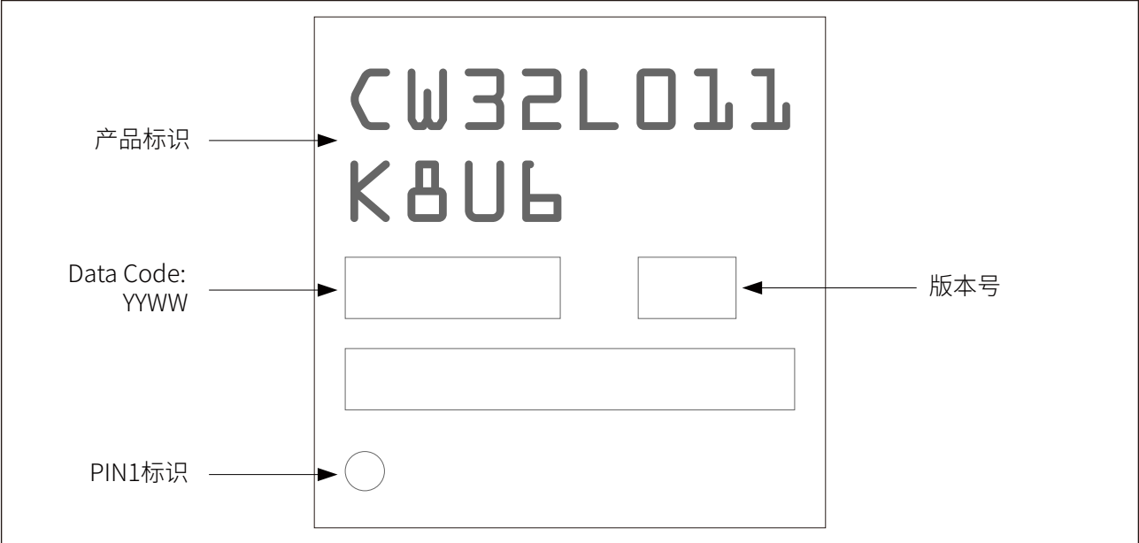
图 8-4 QFN32（4mm×4mm）顶部标记示例
