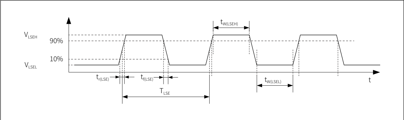
图 7-6 低速外部时钟源交流时序
