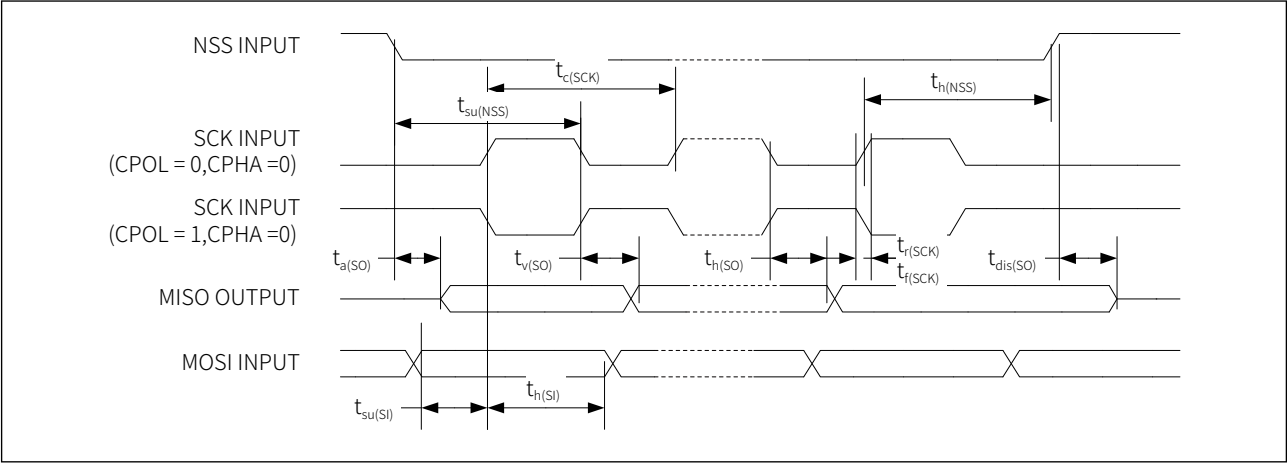
图 7-11 SPI 时序图-从模式 CPHA=0
