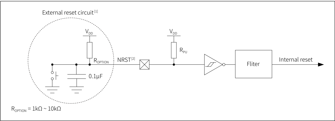
图 7-8 推荐的 NRST 引脚电路
