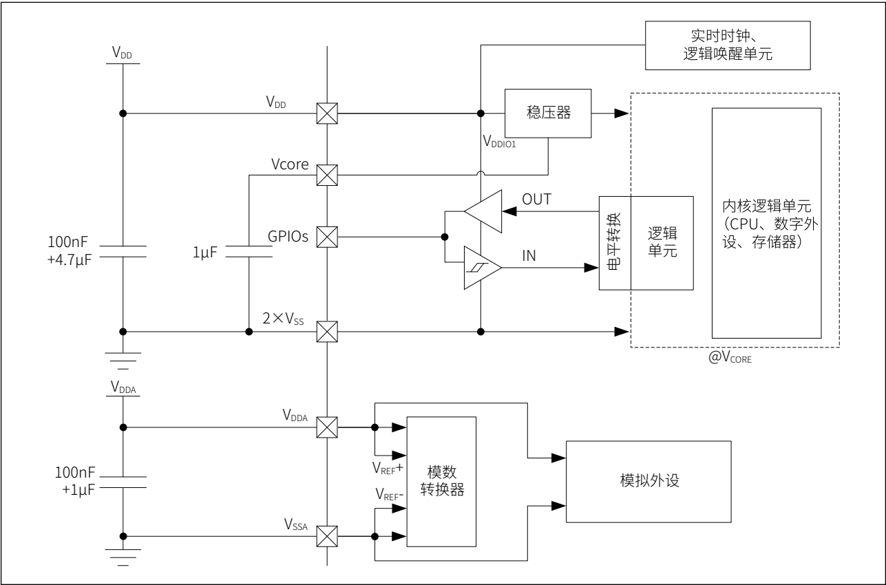
图 7-3 电源系统
