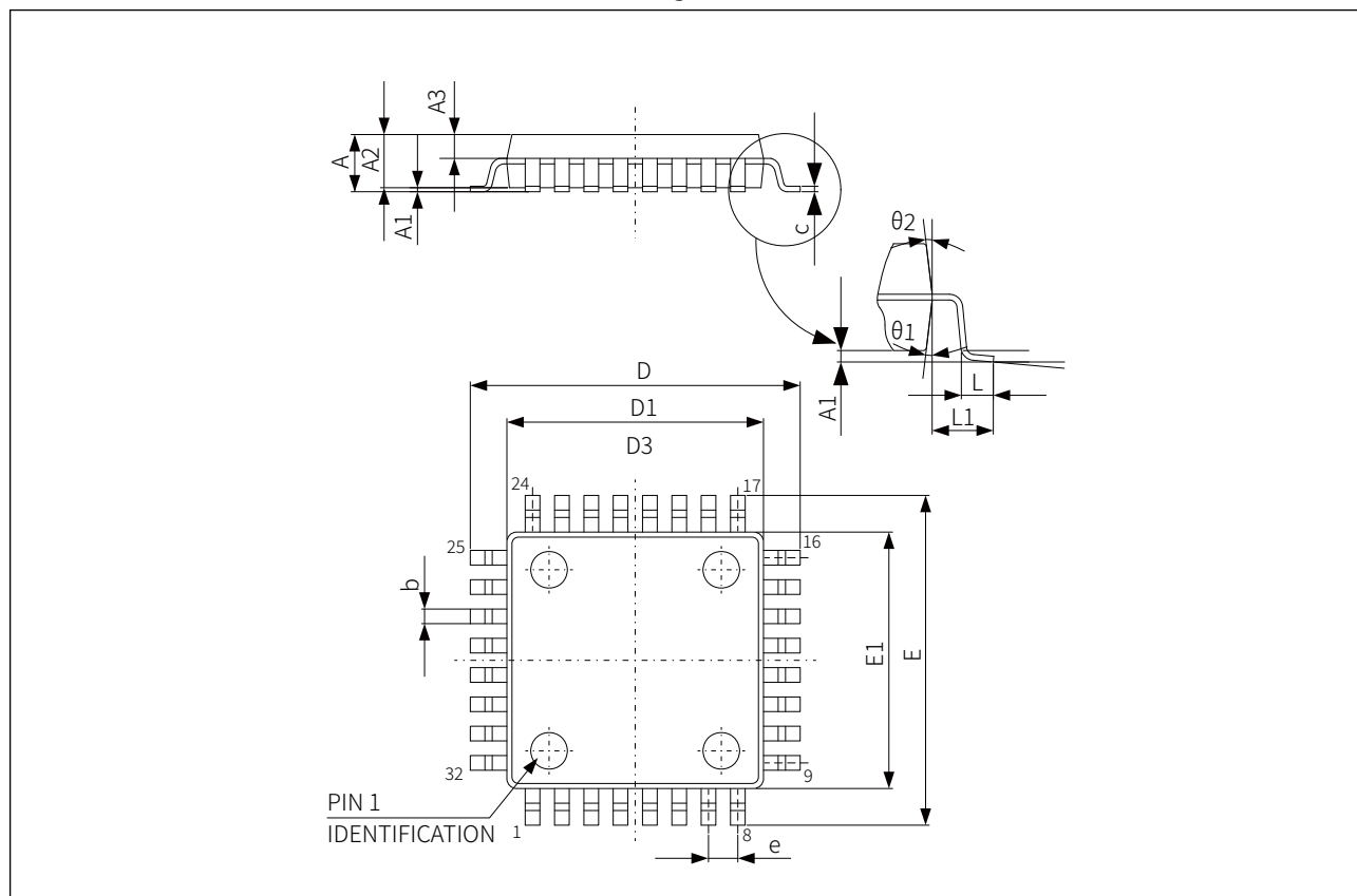
图 8-1 LQFP32 引线
