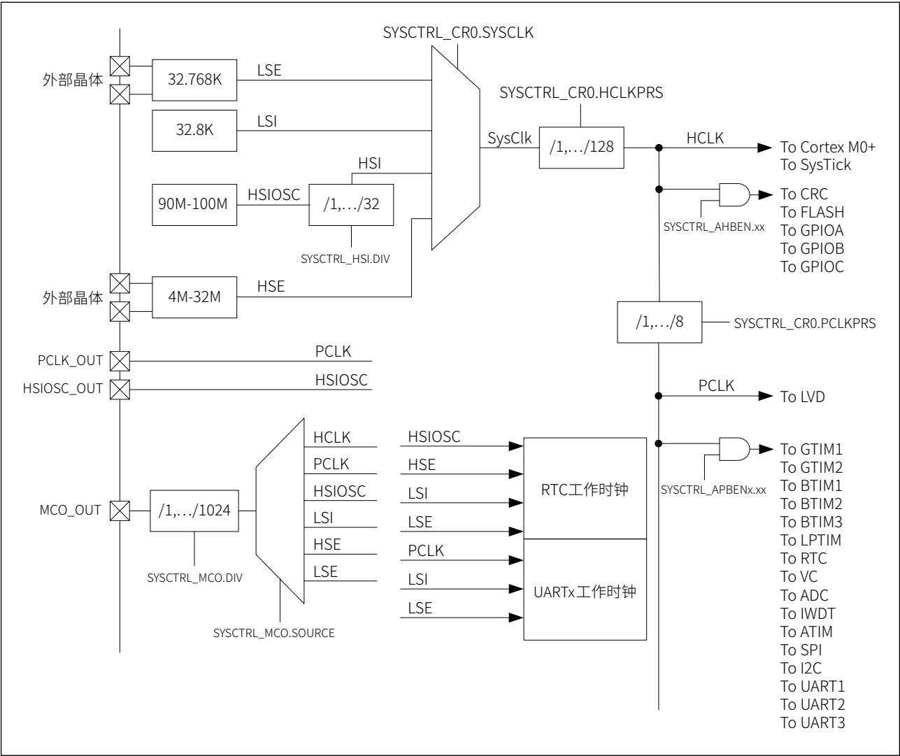
图 4-1 CW32L011 的时钟树
