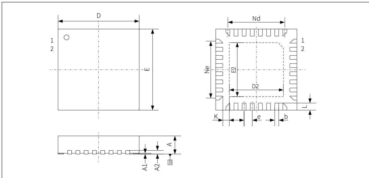
图 8-3 QFN32 (4mm×4mm) 引线
