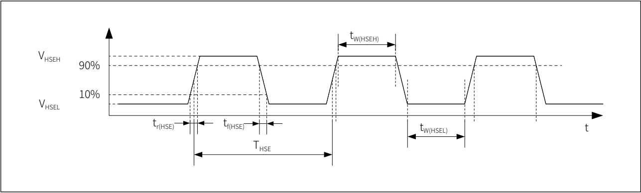
图 7-5 高速外部时钟源交流时序
