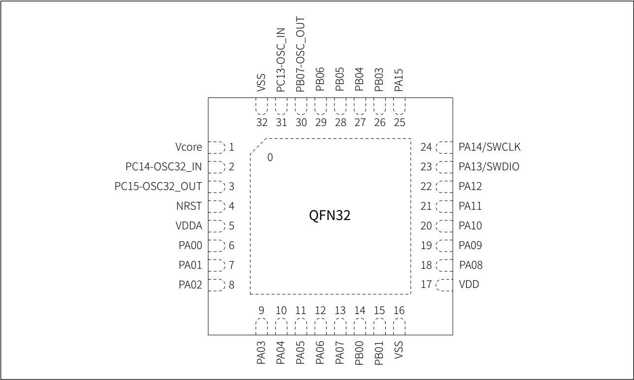
图 5-2 QFN32 封装引脚图（顶视图）
