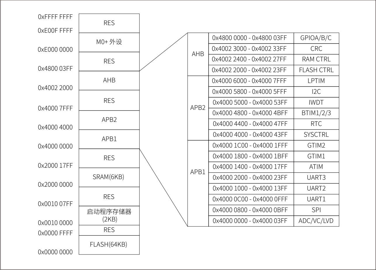
图 6-1 CW32L011 的内部地址镜像
