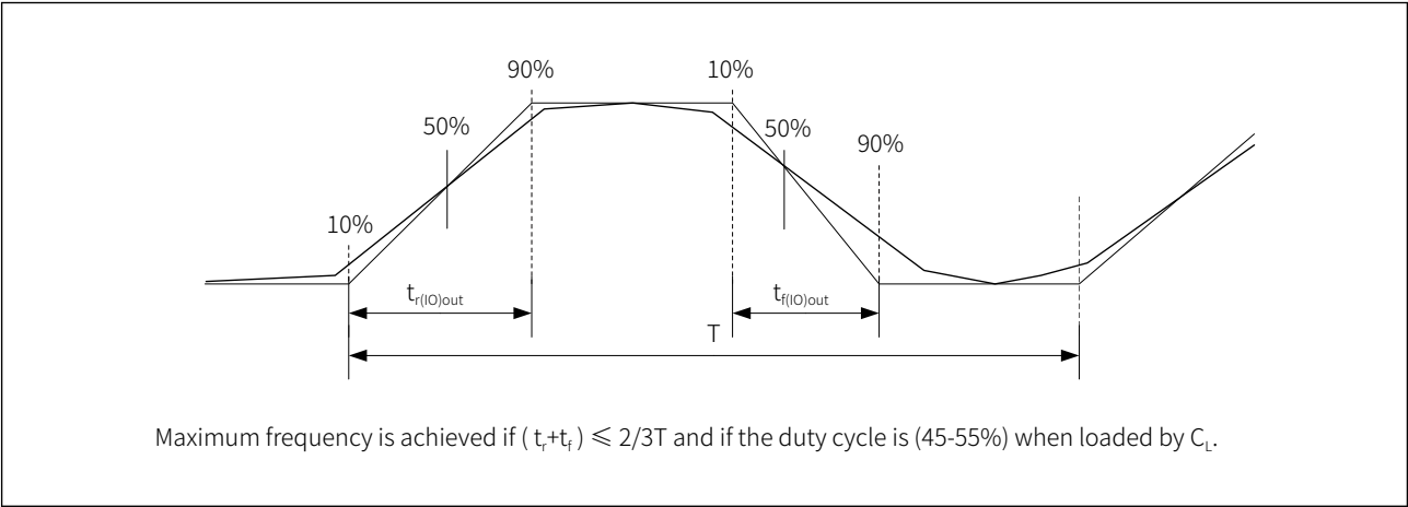
图 7-7 I/O 口交流特性定义
