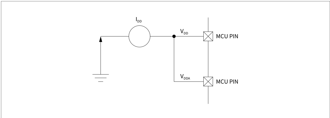
图 7-4 测试方式
