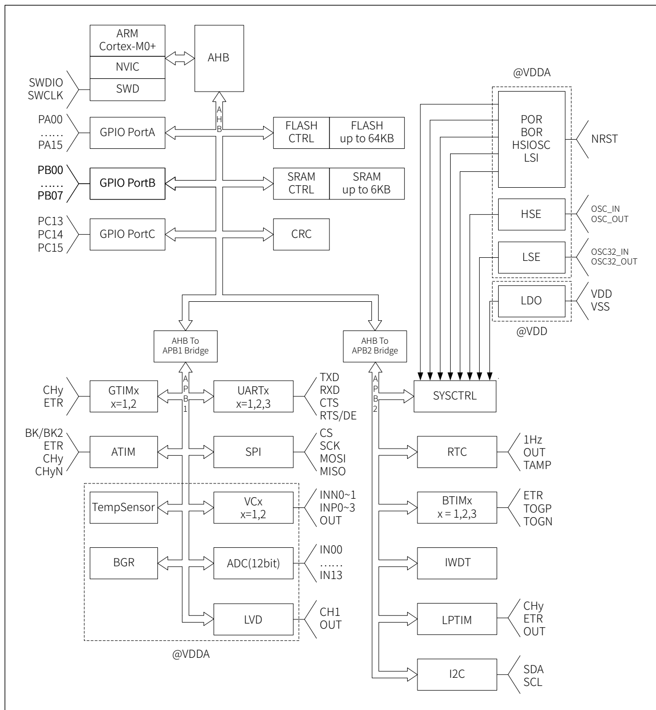
图 3-1 内部框图
