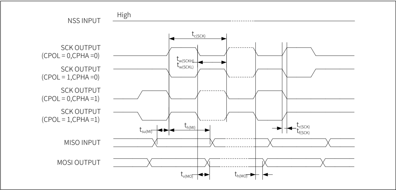
图 7-13 SPI 时序图-主模式
