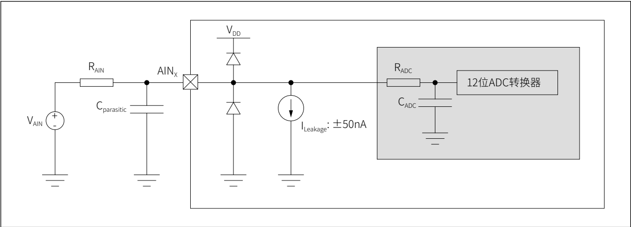
图 7-9 ADC 的典型应用
