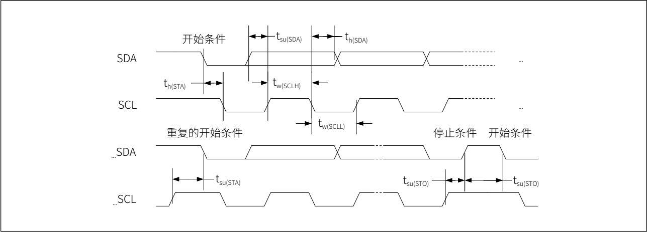
图 7-10 I2C 时序图
