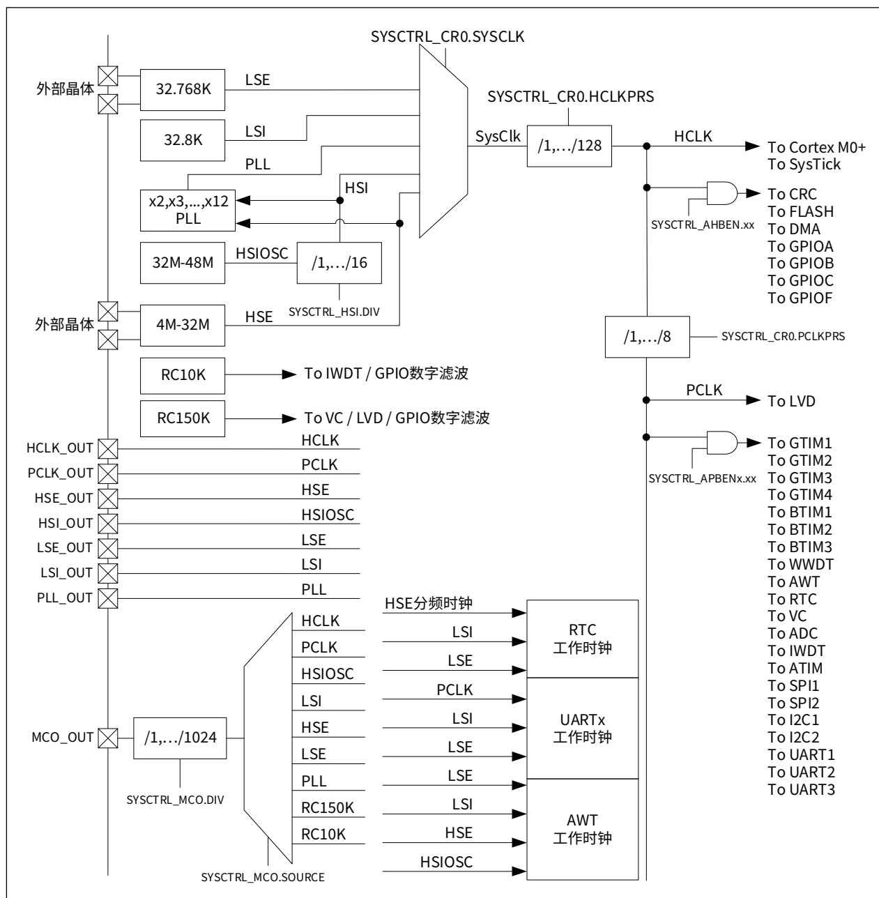
图 4-1 CW32A030 的时钟树
