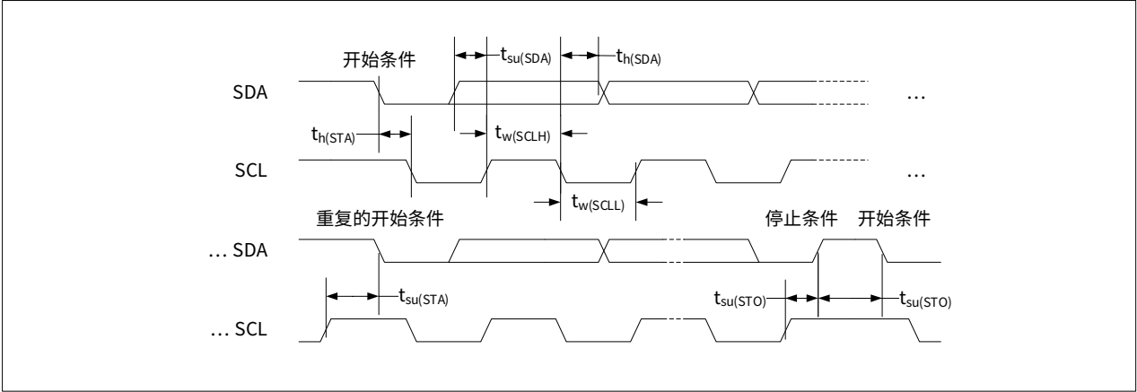
图 7-9 I2C 时序图
