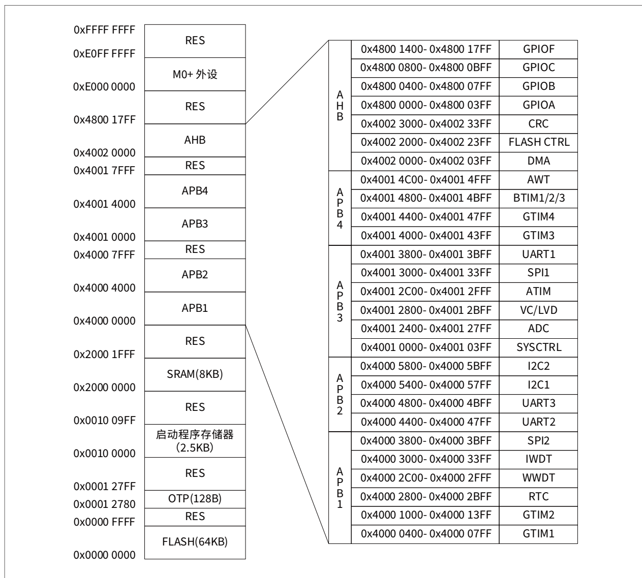
图 6-1 CW32A030 的内部地址镜像
