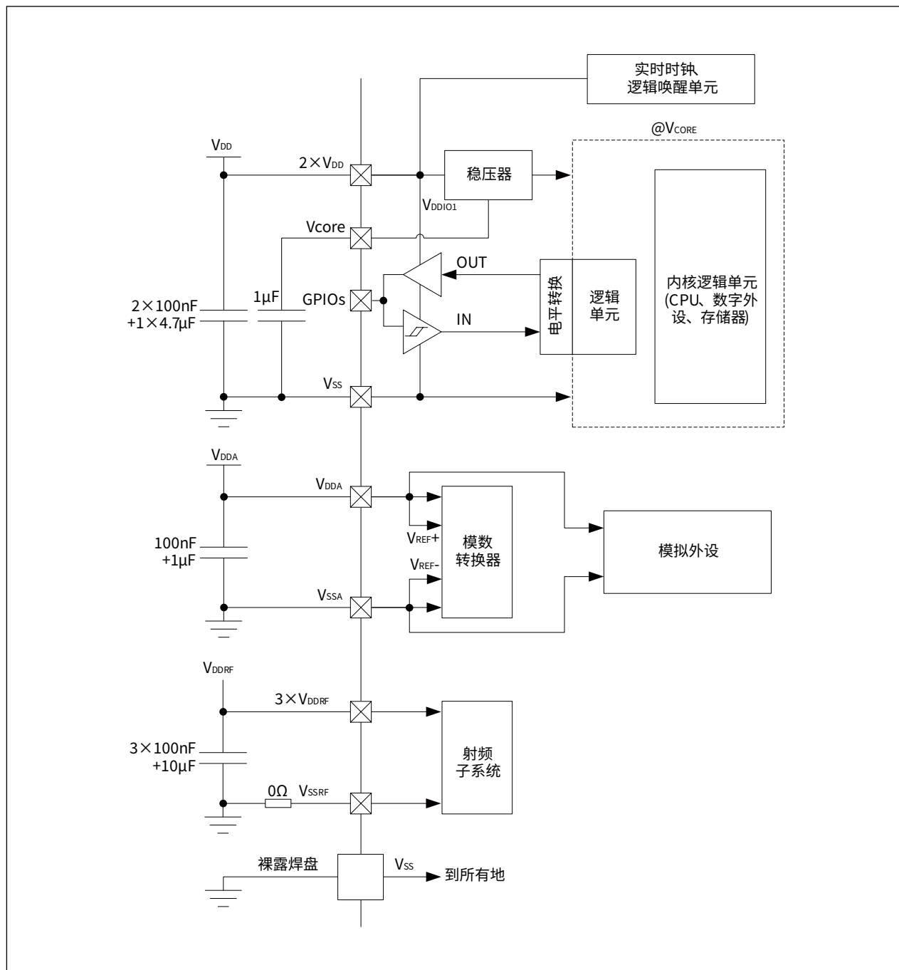
图 7-3 电源系统
