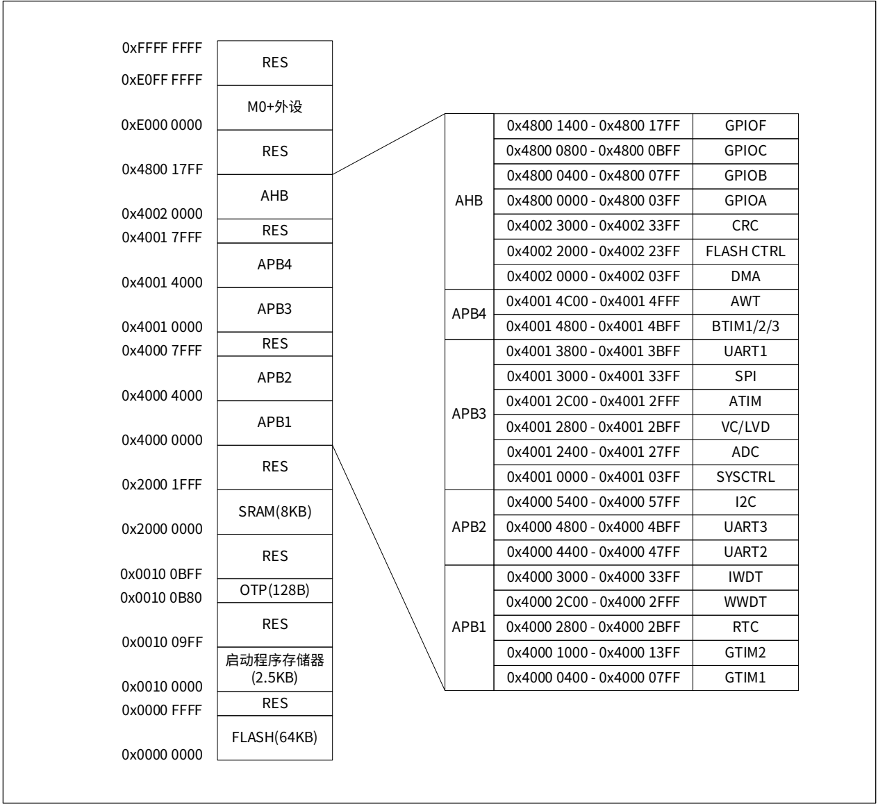
图 6-1 CW32R031 的内部地址镜像
