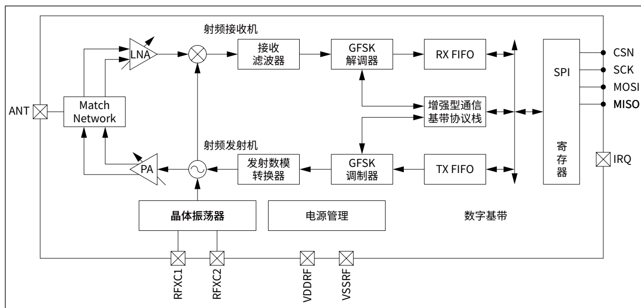
图 4-1 射频前端功能框图
