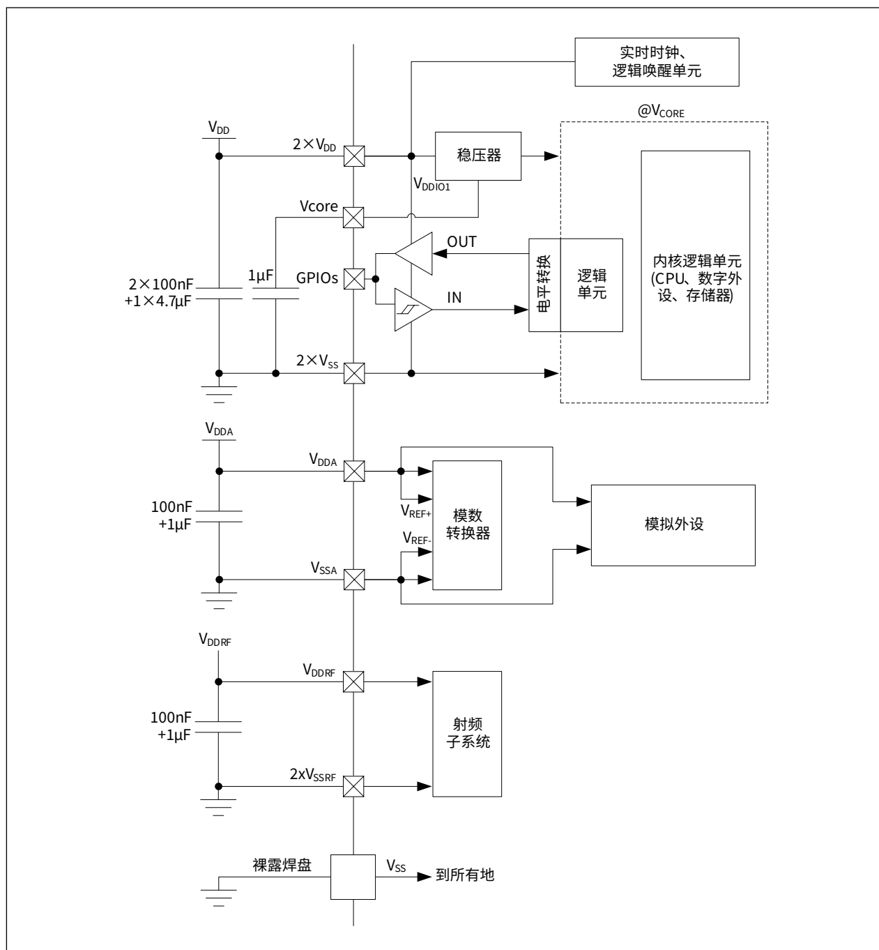
图 7-3 电源系统
