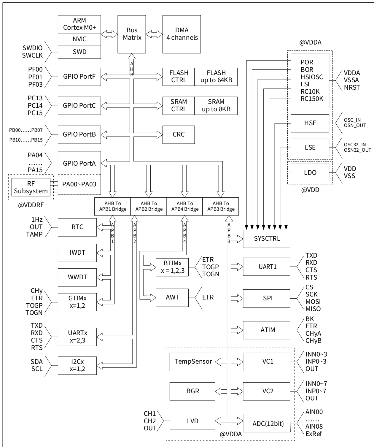
图 3-1 内部框图
