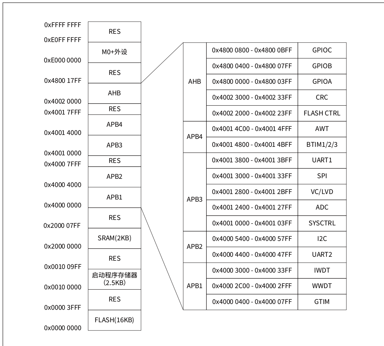
图 6-1 CW32F002 的内部地址镜像
