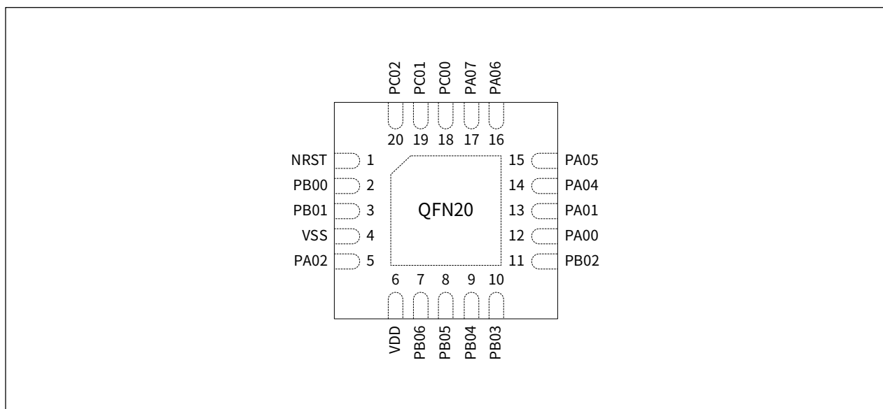
图 5-2 QFN20 封装引脚图（顶视图）
