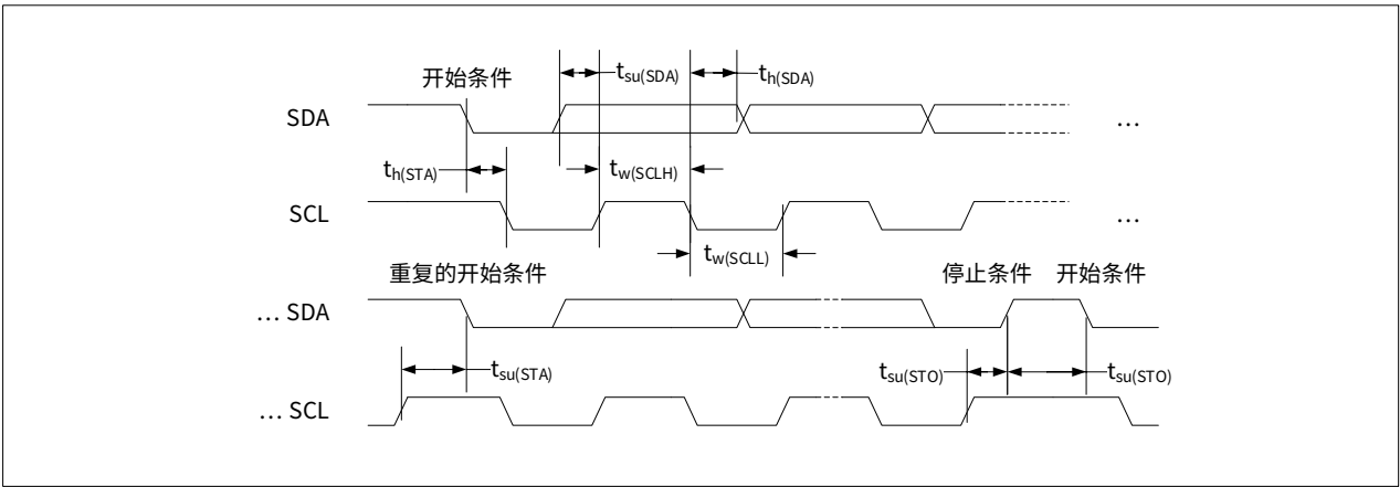
图 7-8 I2C 时序图
