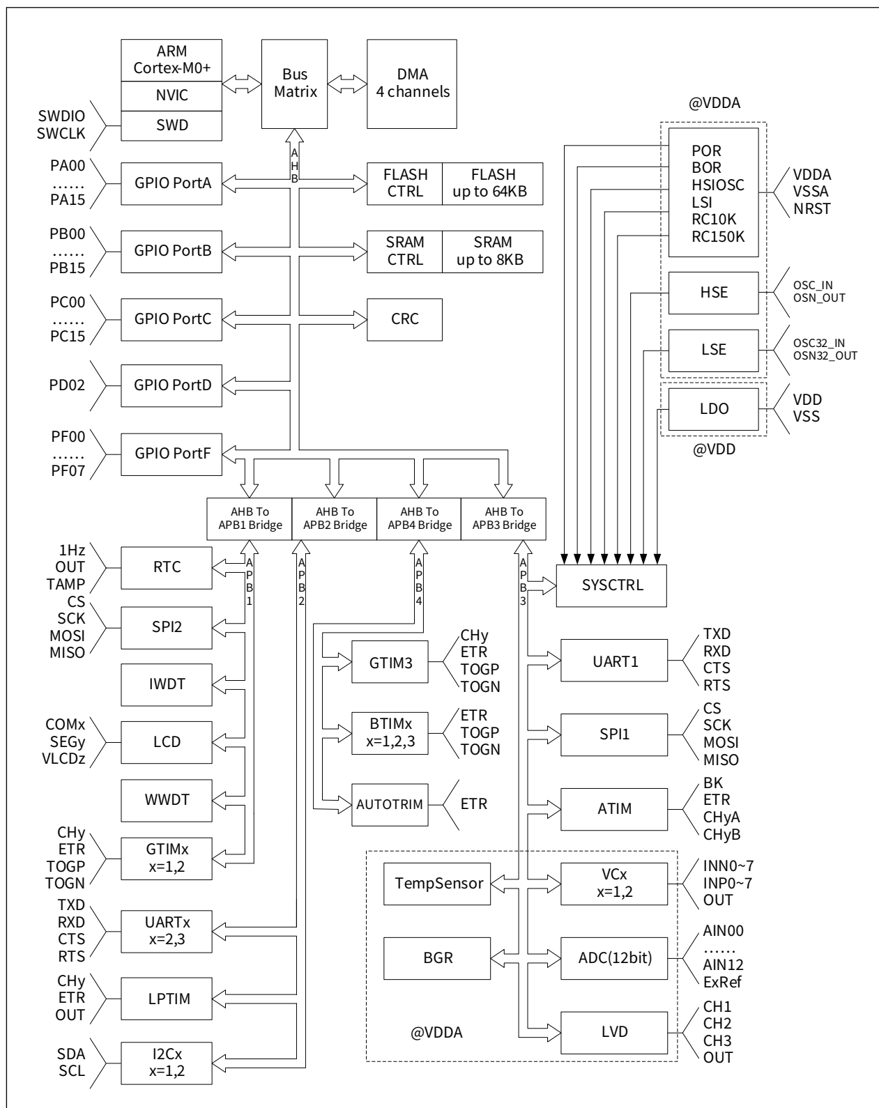
图 3-1 内部框图
