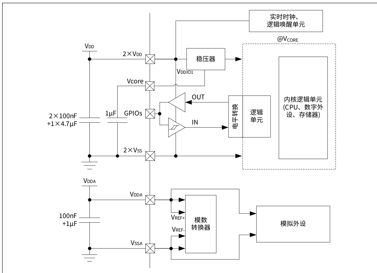
图 7-3 电源系统
