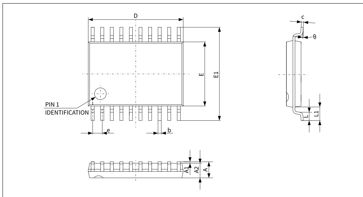
图 8-3 TSSOP20 引线
