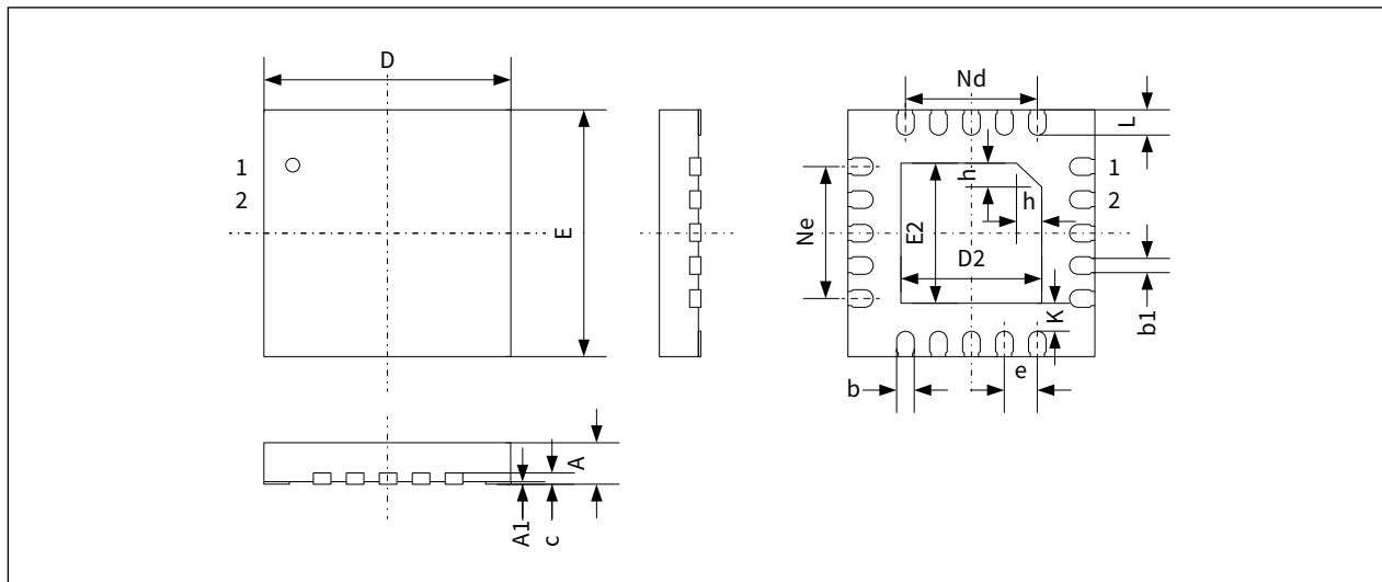
图 8-9 QFN20 引线
