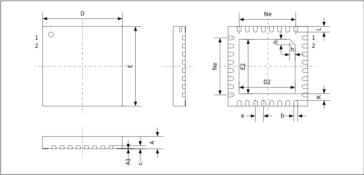
图 8-5 QFN32 (5mm×5mm) 引线
