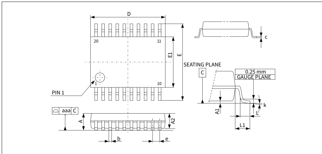
图 8-11 TSSOP20 引线
